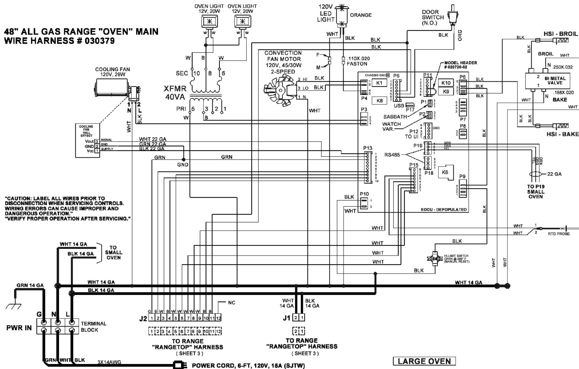
WIRING DIAGRAM, KRG484GD 030180
