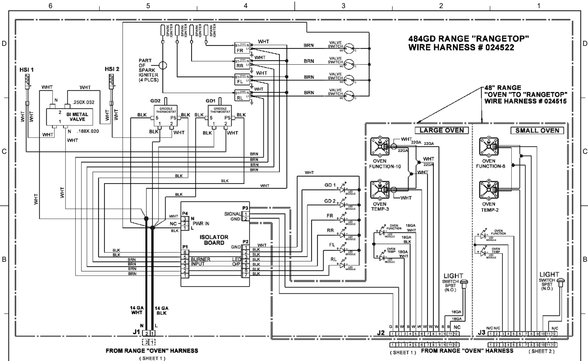
WIRING DIAGRAM, KRG484GD 030180
