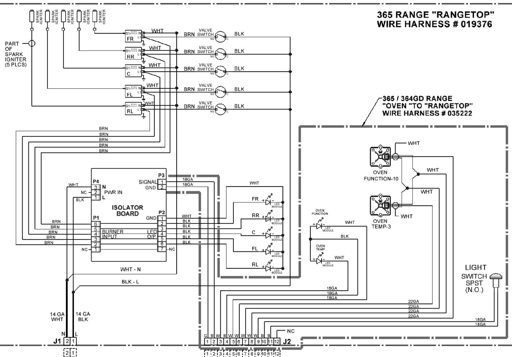
WIRING DIAGRAM, KRD365 018161
