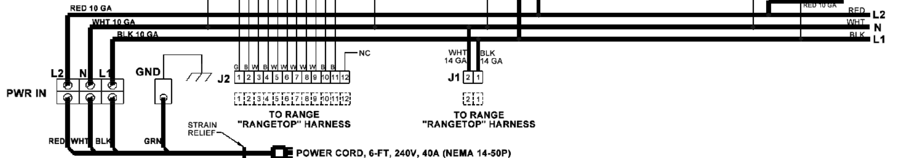
WIRING DIAGRAM, KRD365 018161
