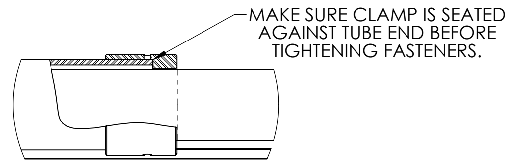
DETAIL A SCALE: 1:2
