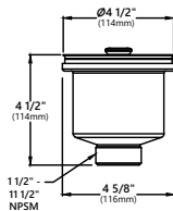
Model # / No de modèle: BST-1 Dimensions / Les dimensions: \varnothing 4 \frac{1}{2}'' \times 4 \frac{1}{2}''
