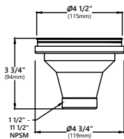
Model # / No de modèle: ST-1 Dimensions / Les dimensions: \varnothing 4 \frac{1}{2}'' \times 3 \frac{3}{4}''
