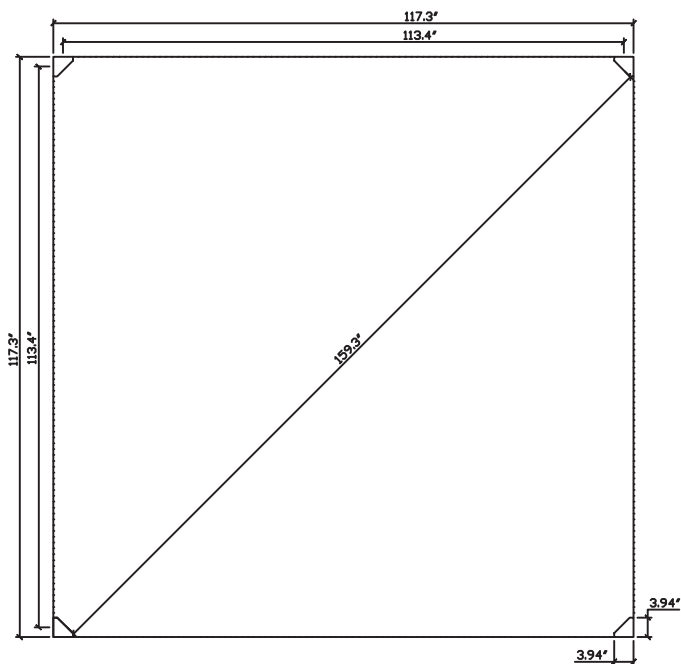
VUE DE LA BASE DE LA STRUCTURE VIEW OF STRUCTURE BASE
