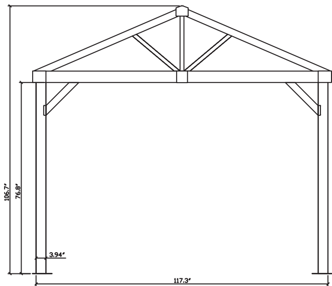
VUE DE CÔTÉ | SIDE VIEW
