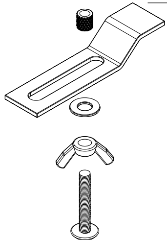
Kit for Drop-In Installation / Trousse d'installation en surface
