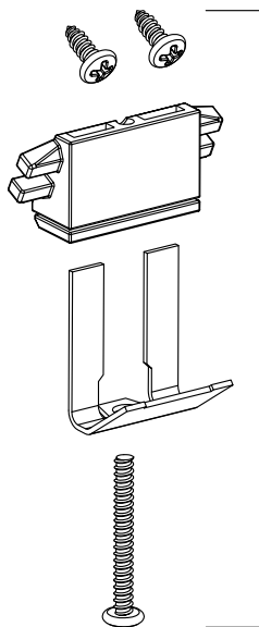
Kit for Drop-In Installation / Trousse d'installation en surface
