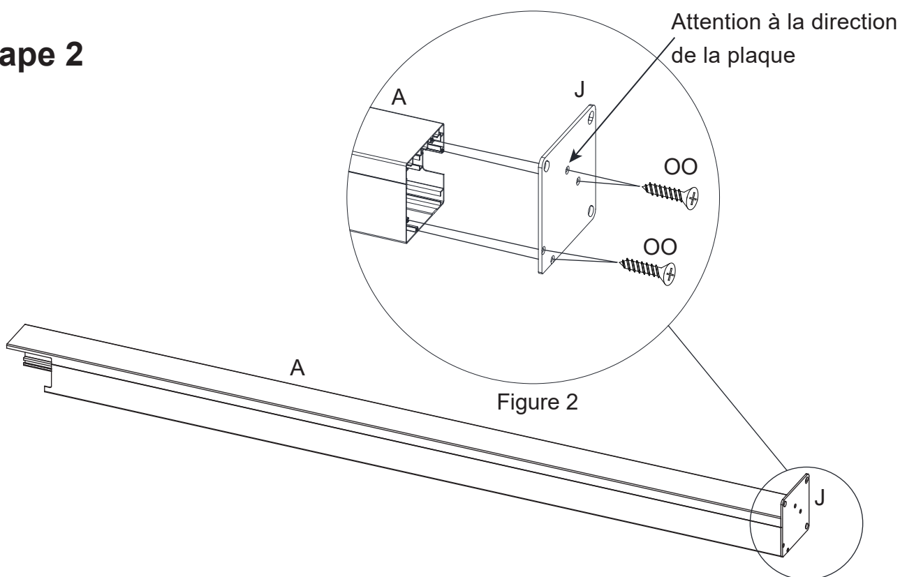
Figure 2. Faites attention à la direction de la plaque d'ancrage. Connectez la plaque d'ancrage (J) à la poutre en coin (A) et fixez-les à l'aide des boulons (OO).
