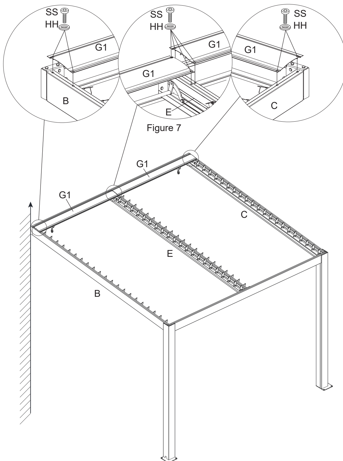
Figure 7. Connectez la plaque de recouvrement (G1) aux traverses (B/C/E) à l'aide des boulons (SS) et des rondelles (HH).
