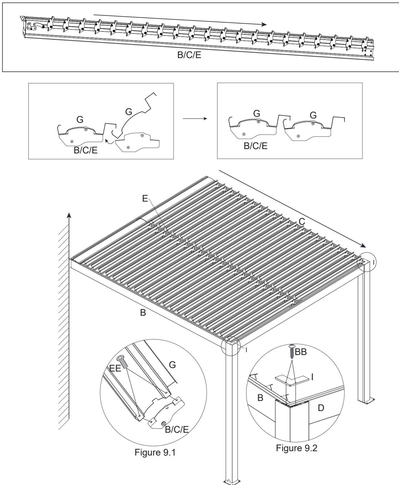
Figure 9.1. Assemblez les autres volets dans le sens des flèches et fixez-les avec les boulons (EE). Figure 9.2. Connectez le capuchon de poutre avec la poutre en coin (A) et fixez-le à l'aide des boulons (BB).
