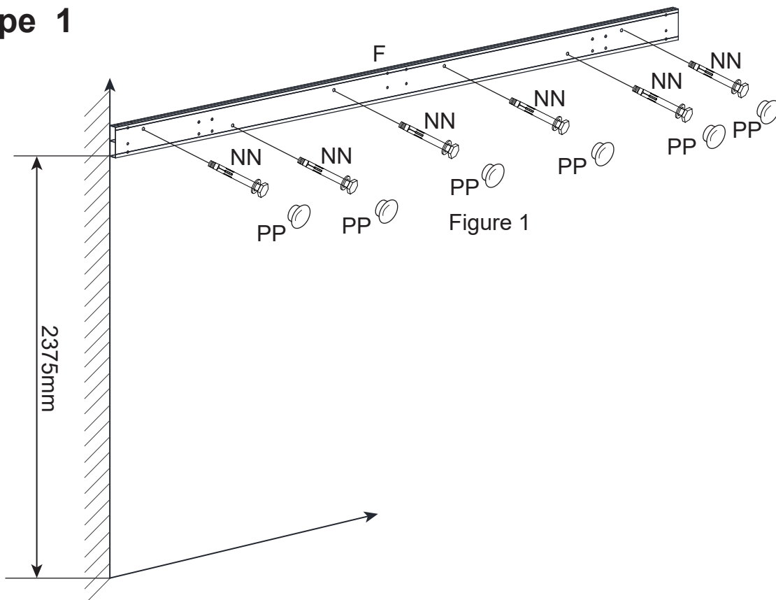
Figure 1. Ajustez la hauteur de la traverse arrière (F) 237.5cm en mesurant à partir du sol et fixez-la au mur à l'aide des boulons (NN). Couvrez ensuite les trous avec les capuchons en plastique (PP).
