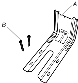
A. Bride antibascullement B. Vis n° 12 x 1 5/8" (2)
