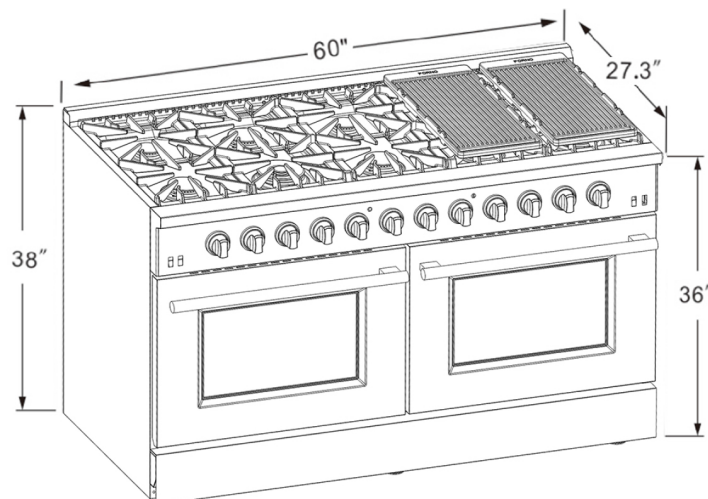
Model: FFSGS6244-60
