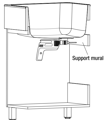
Coupe transversale de l'armoire Certains composants ont été retirés pour plus de clarté
