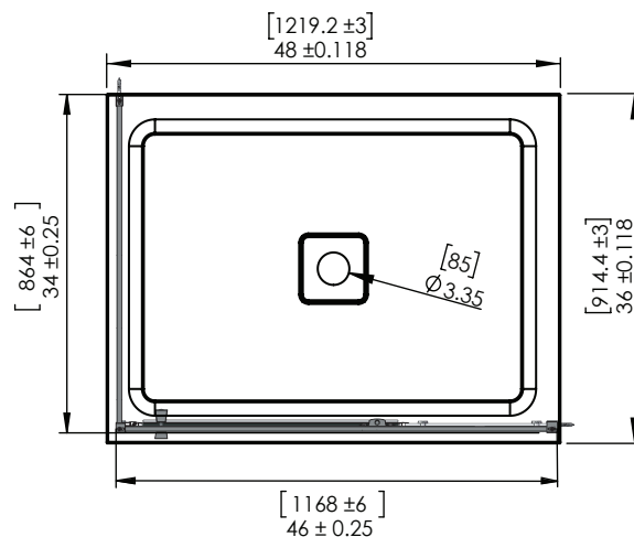
TOP VIEW VUE DU HAUT
