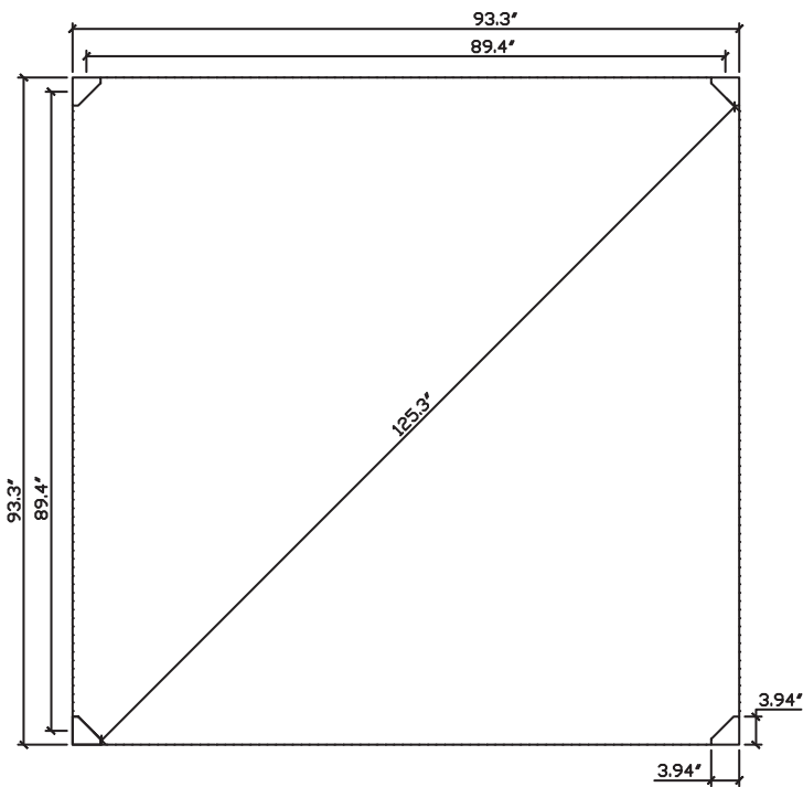
VUE DE LA BASE DE LA STRUCTURE VIEW OF STRUCTURE BASE
