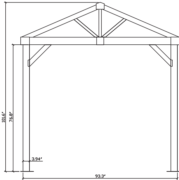
VUE DE CÔTÉ | SIDE VIEW
