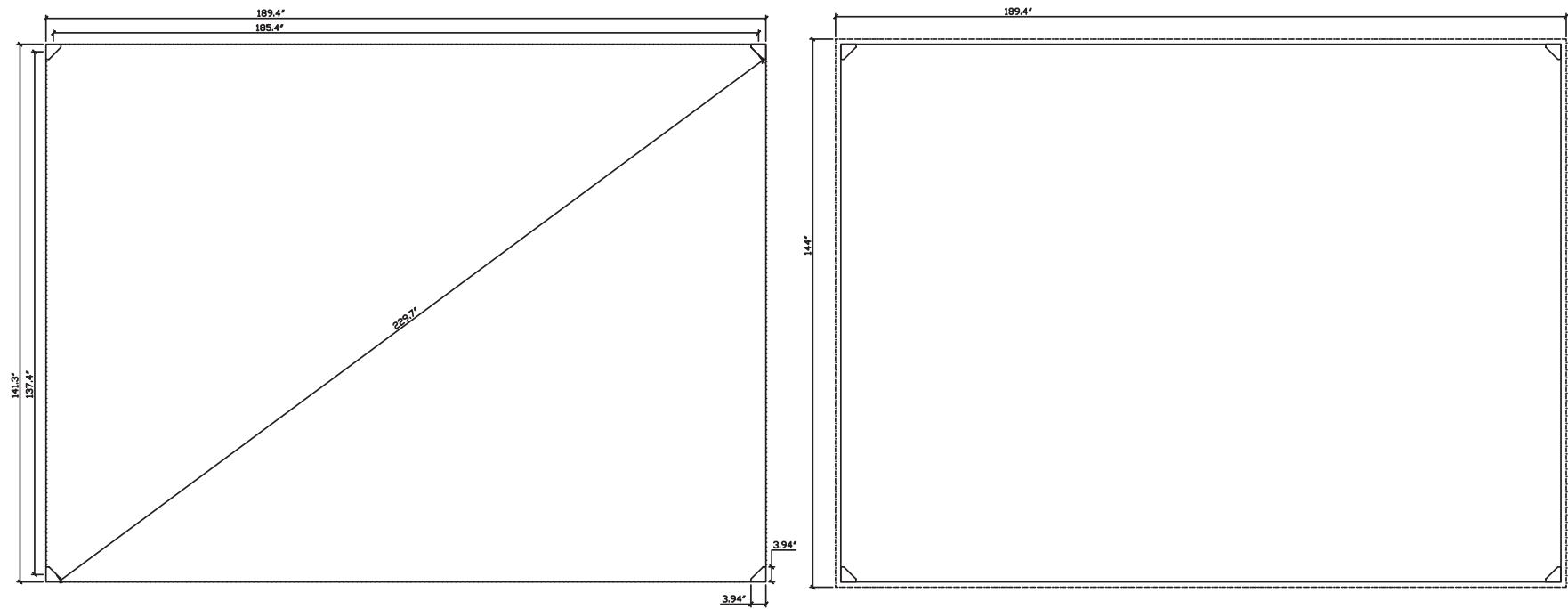
VUE DE LA BASE DE LA STRUCTURE VIEW OF STRUCTURE BASE
