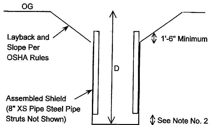
TYP EXC SECTION
