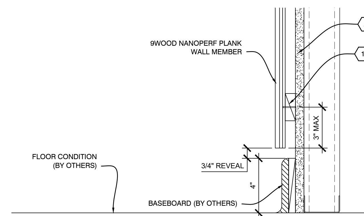
A4 SECTION - FLOOR PERIMETER SCALE: 1/4" = 1"
