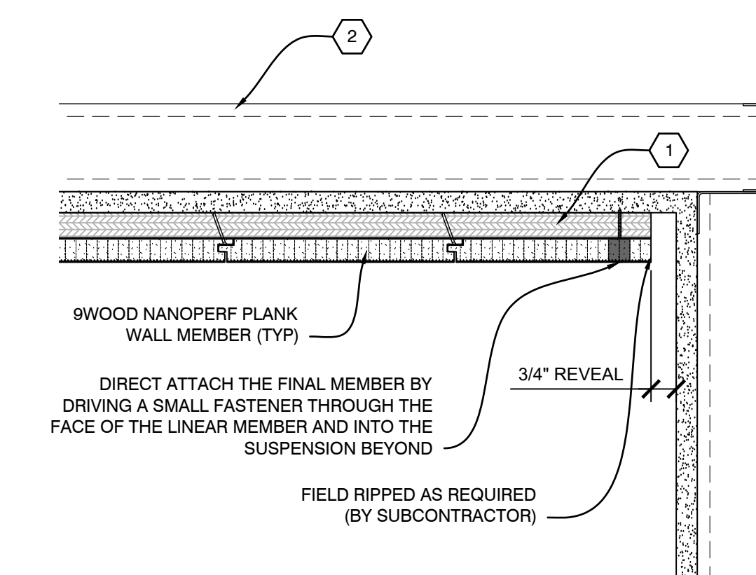
A3 PLAN VIEW - PERIMETER SCALE: 1/4" = 1"
