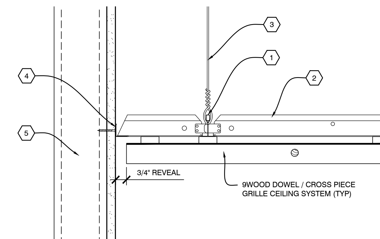
A1 SECTION - PERIMETER SCALE: 1/4" = 1"
