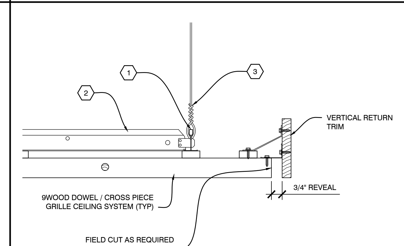
A4 SECTION - PERIMETER SCALE: 1/4" = 1'
