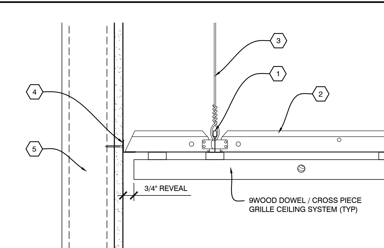
A1 SECTION - PERIMETER SCALE: 1/4" = 1'
