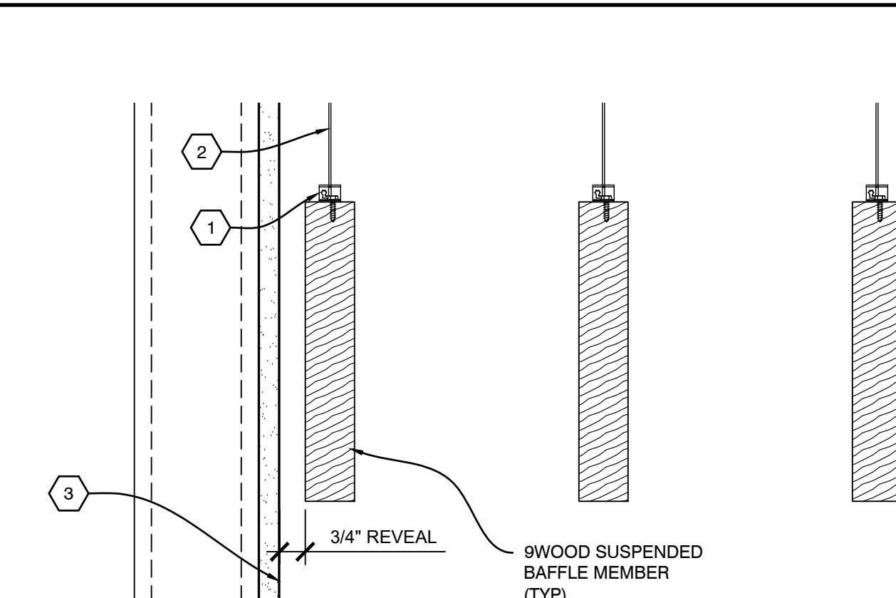
A1 SECTION - PERIMETER SCALE: 1/4" = 1'
