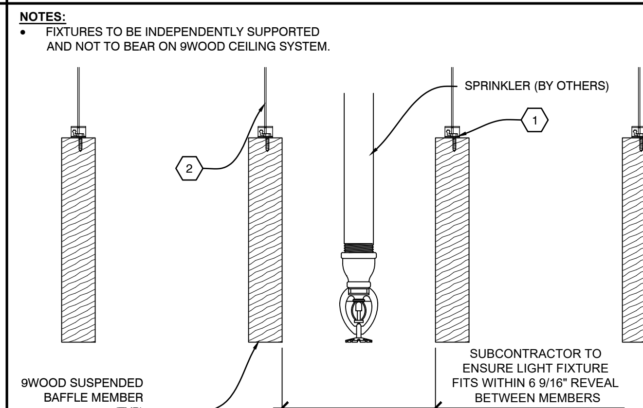
A3 SECTION - SPRINKLER SCALE: 1/4" = 1'
