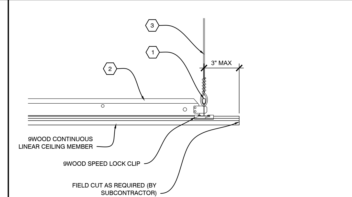
A4 SECTION - PERIMETER SCALE: 1/4" = 1"
