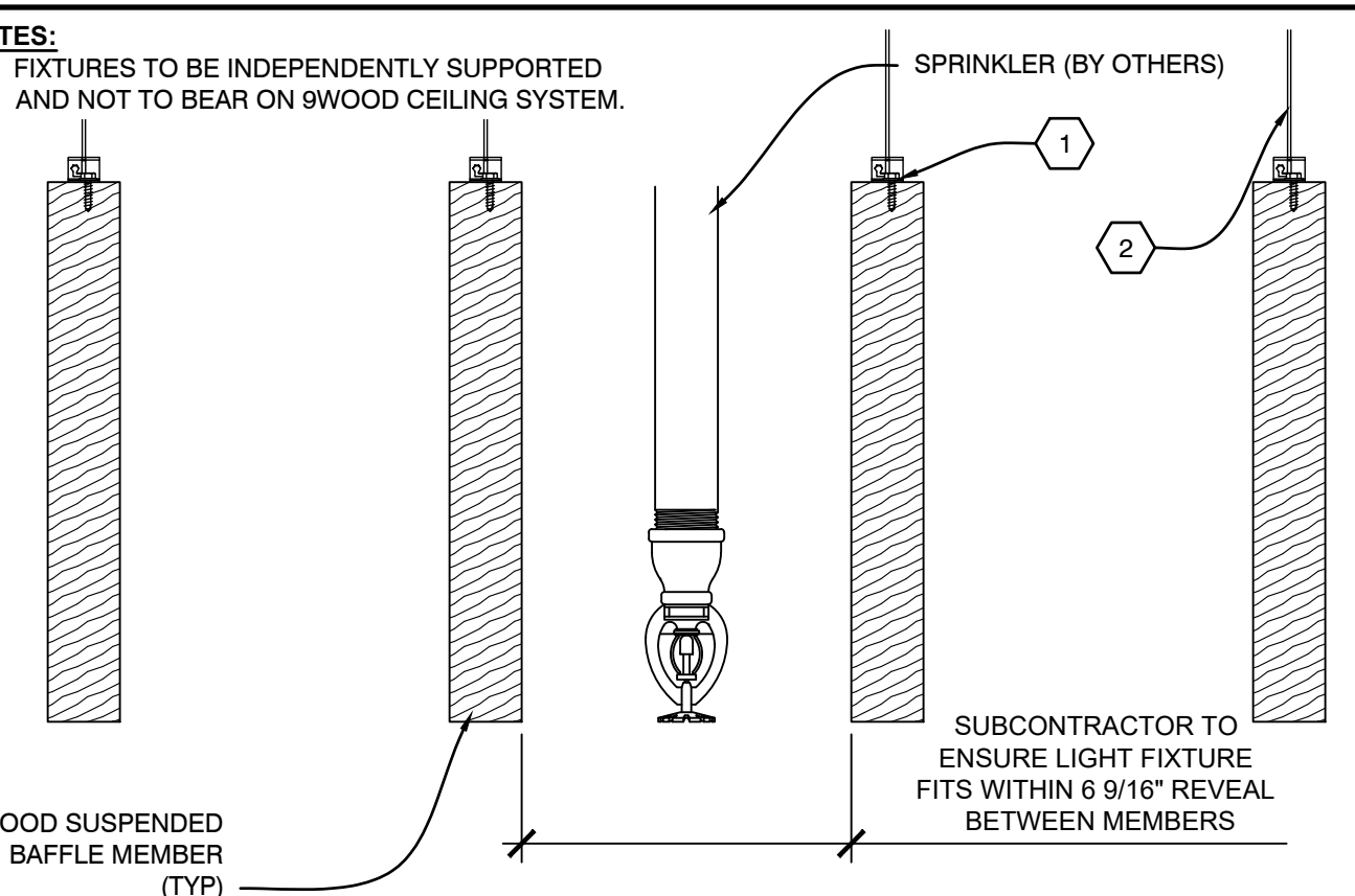
A3 SECTION - SPRINKLER SCALE: 1/4" = 1"
