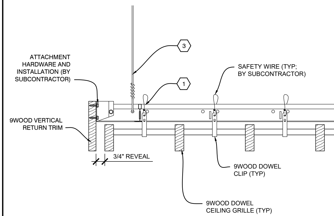
B2 SECTION - PERIMETER SCALE: 1/4" = 1'
