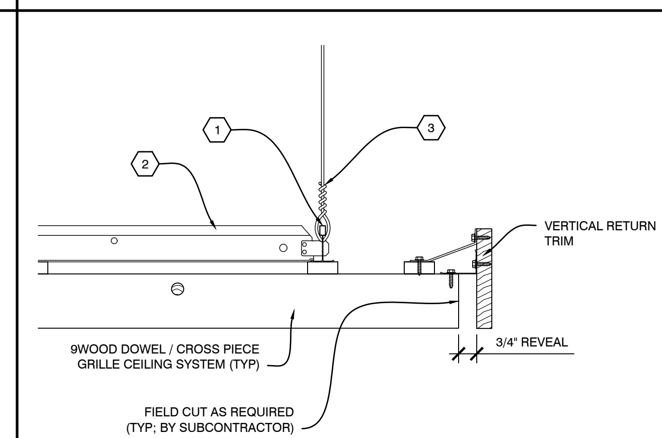
A4 SECTION - PERIMETER SCALE: 1/4" = 1'
