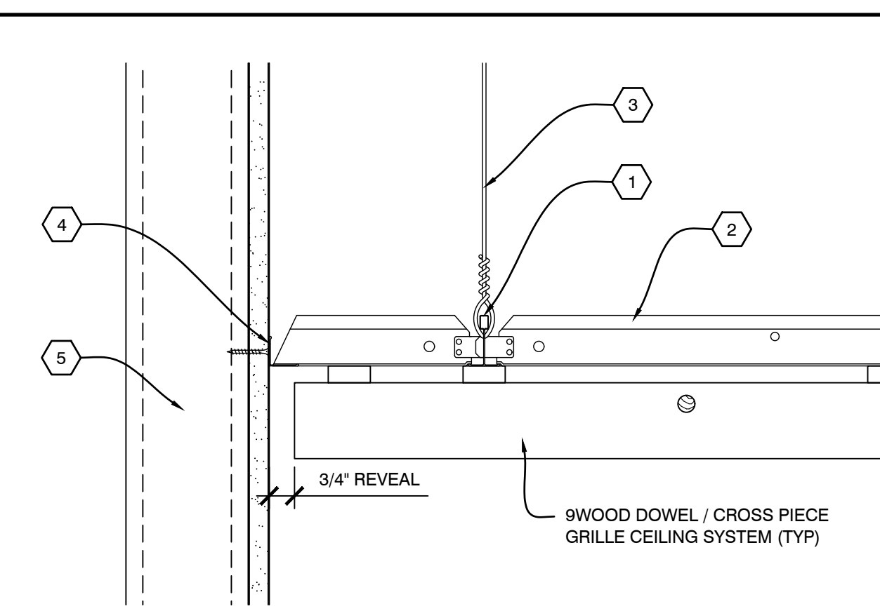
A1 SECTION - PERIMETER SCALE: 1/4" = 1'
