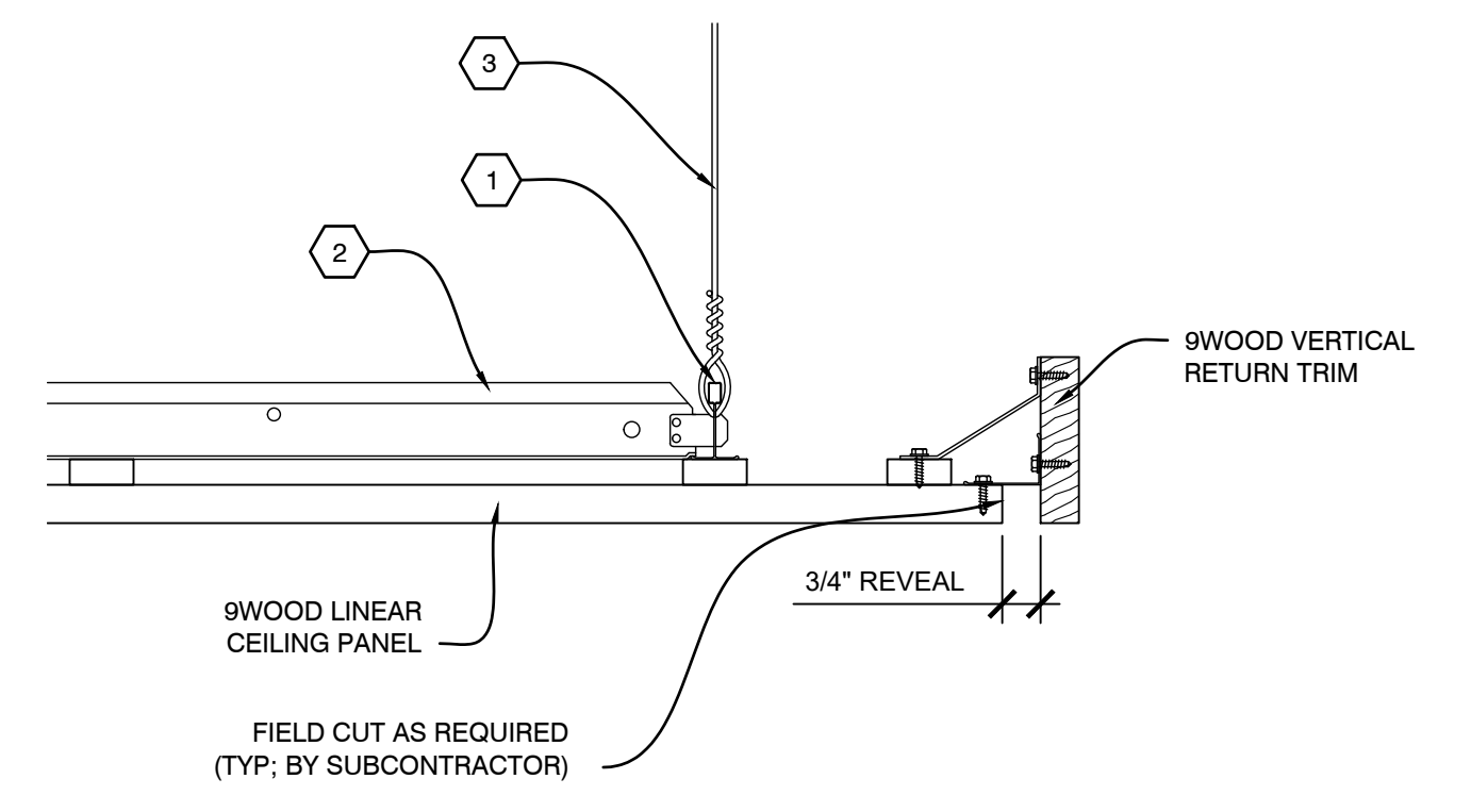
A4 SECTION - PERIMETER SCALE: 1/4" = 1"
