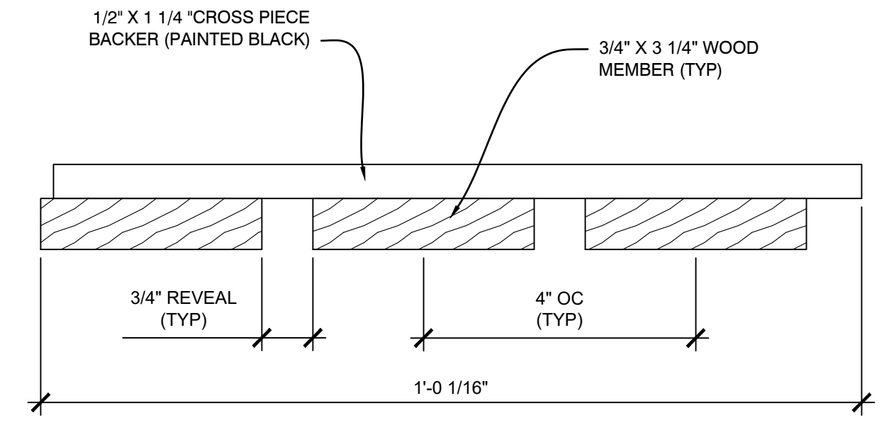
C3 SECTION - LINEAR CEILING PANEL SCALE: 1/2" = 1"
