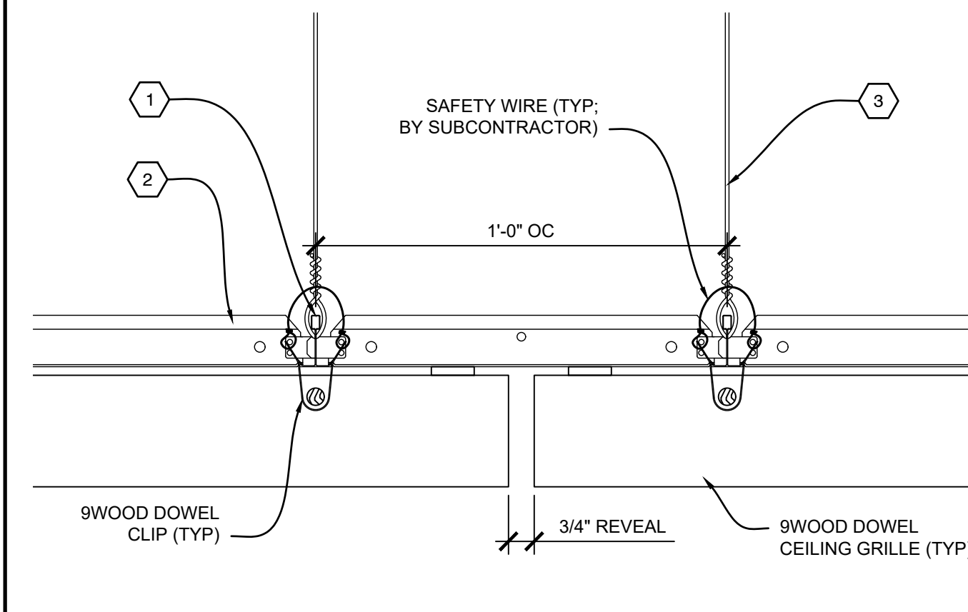
A3 SECTION - REVEAL SCALE: 1/4" = 1"
