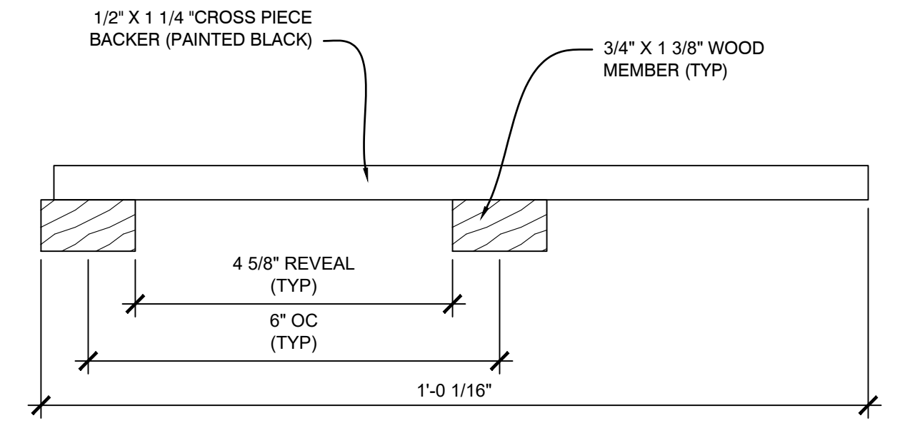
C3 SECTION - LINEAR CEILING PANEL SCALE: 1/2" = 1'
