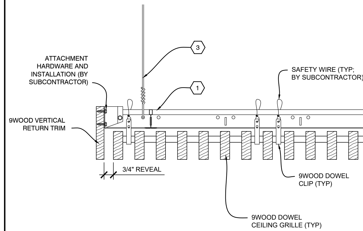
B2 SECTION - PERIMETER SCALE: 1/4" = 1'
