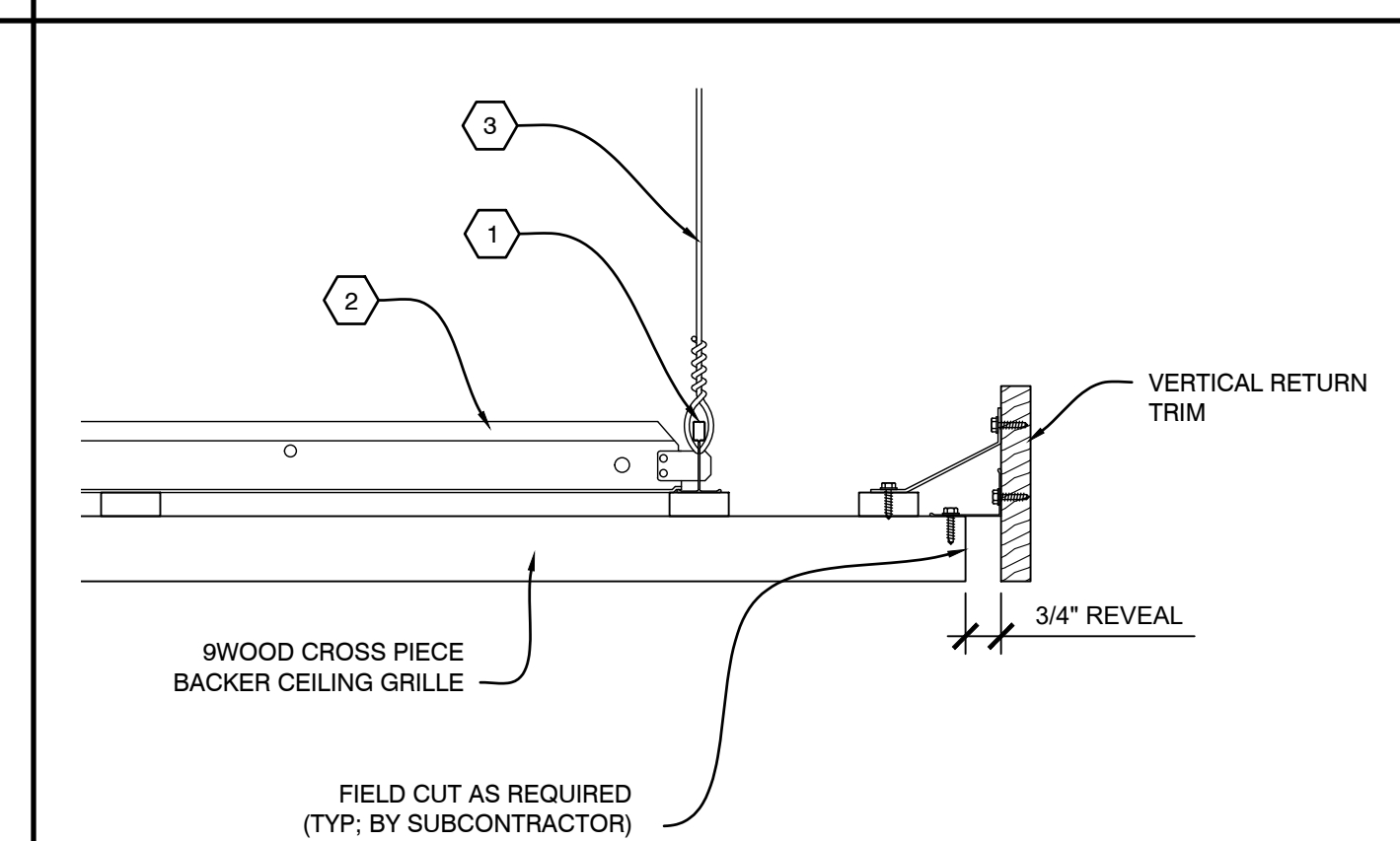
A4 SECTION - PERIMETER SCALE: 1/4" = 1'
