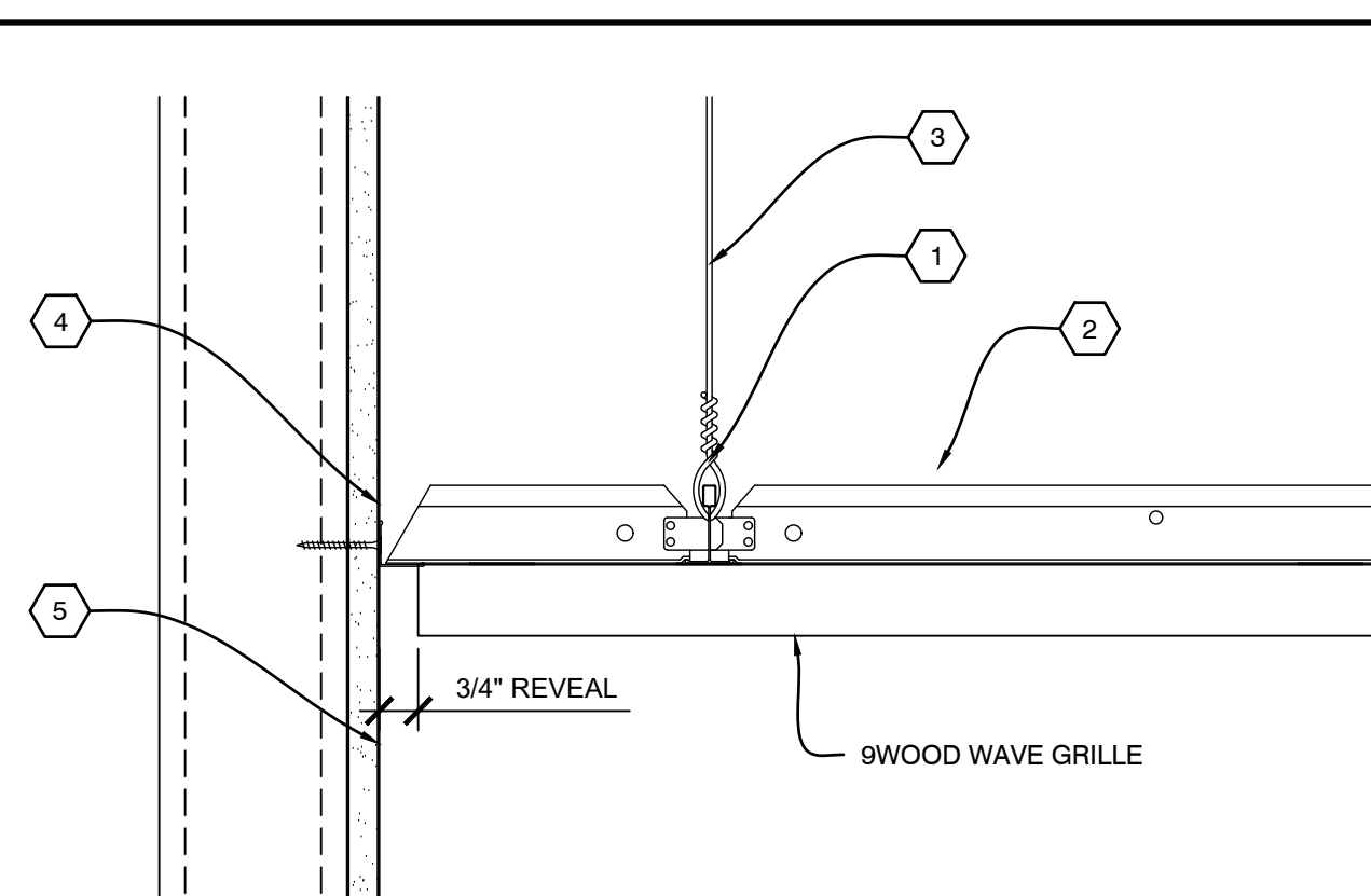
A1 SECTION - PERIMETER
