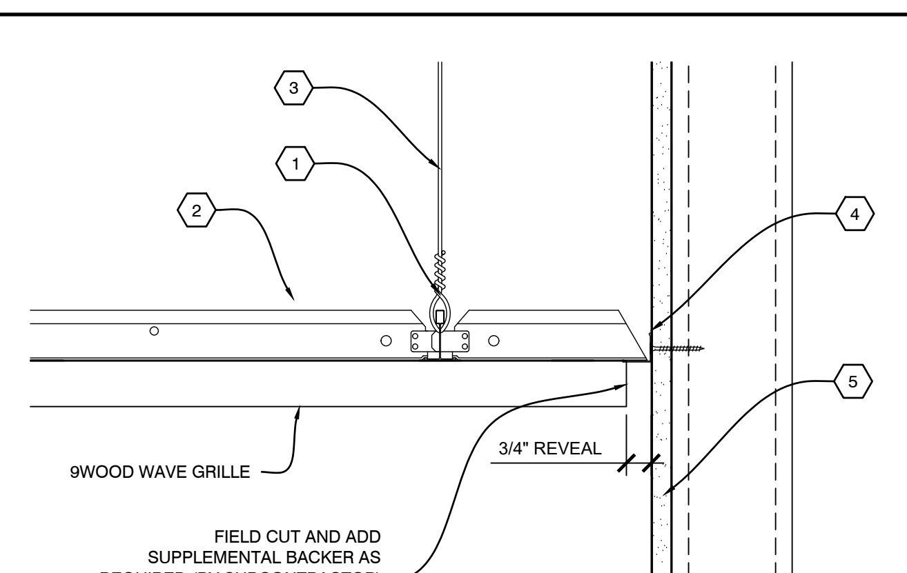
A4 SECTION - PERIMETER
