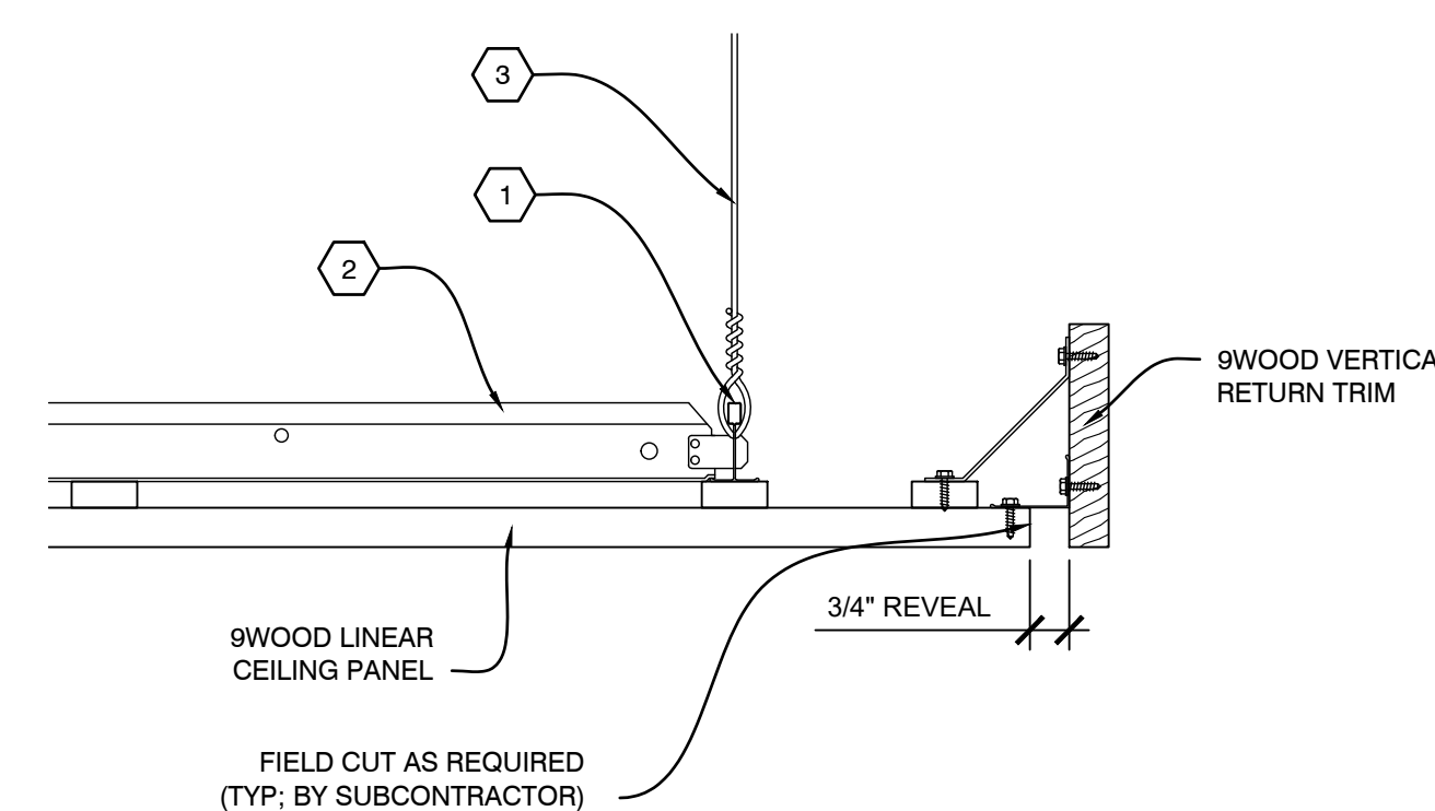
A4 SECTION - PERIMETER SCALE: 1/4" = 1'
