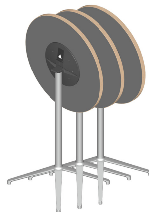
Nested Tables
