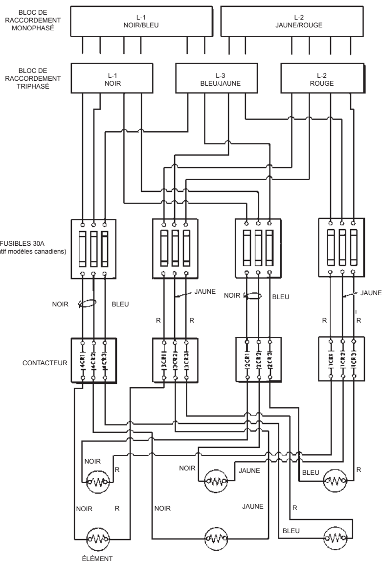
SIX ÉLÉMENTS - MONOPHASÉ ET TRIPHASÉ
