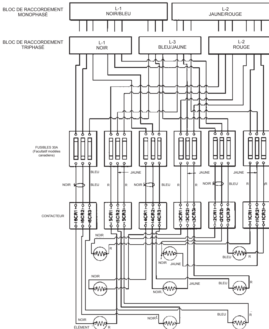
NEUF ÉLÉMENTS - MONOPHASÉ ET TRIPHASÉ
