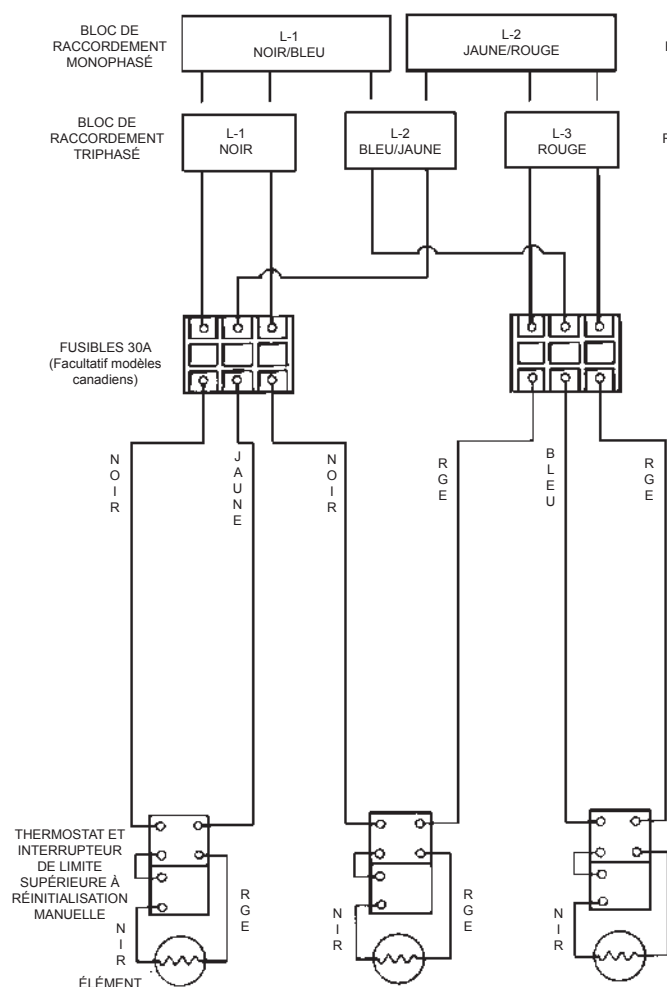
TROIS ÉLÉMENTS - MONOPHASÉ ET TRIPHASÉ
