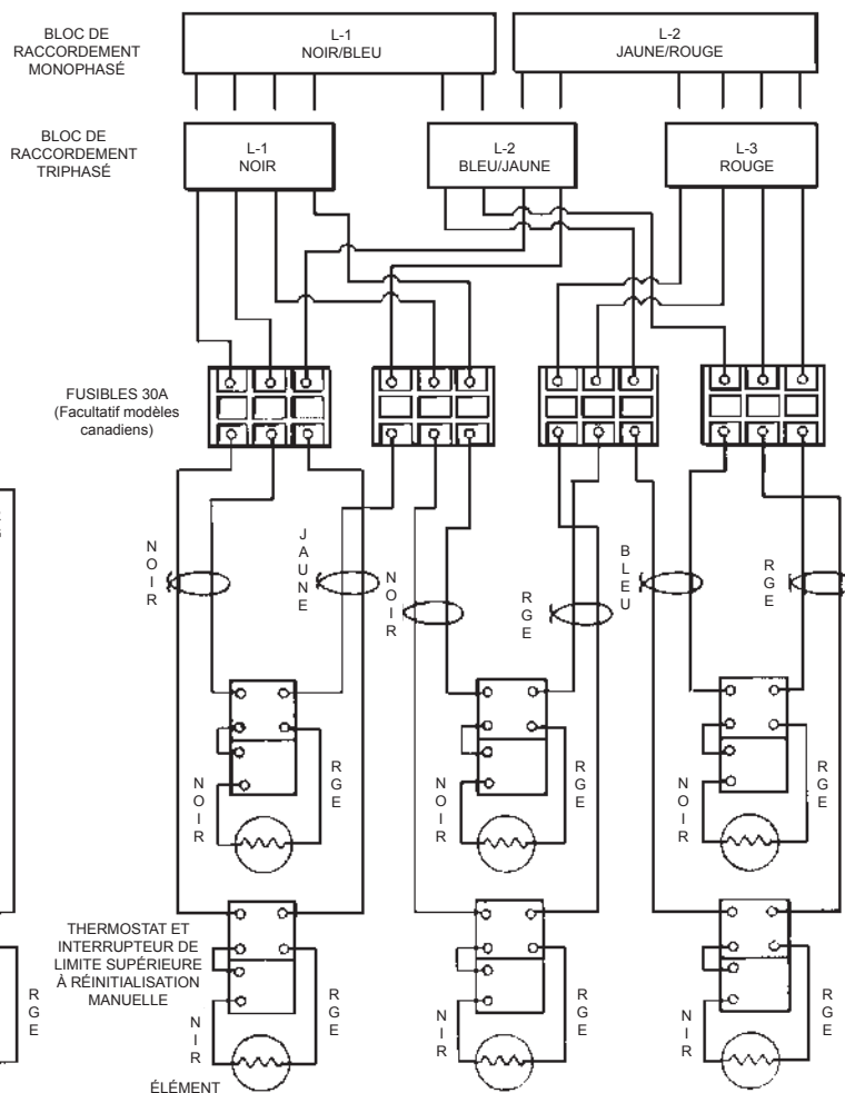
SIX ÉLÉMENTS - MONOPHASÉ ET TRIPHASÉ
