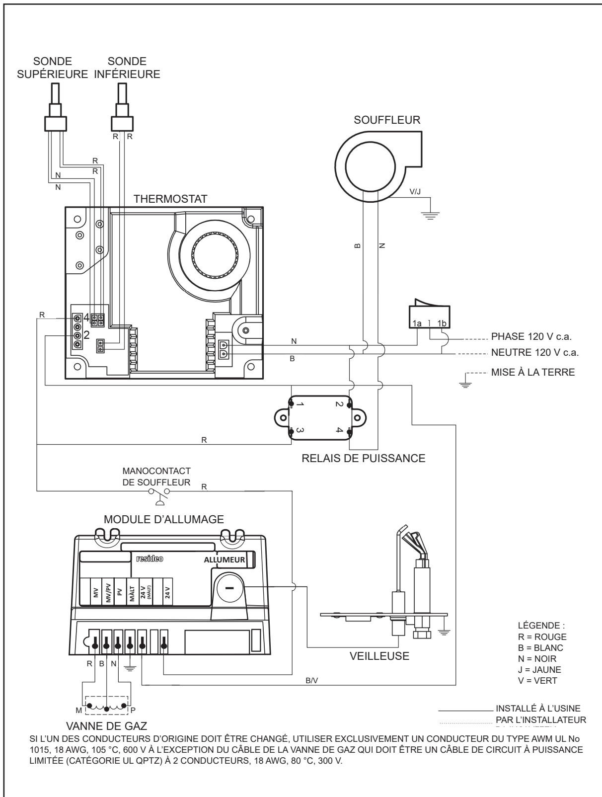
Figure 32. Schéma de câblage
