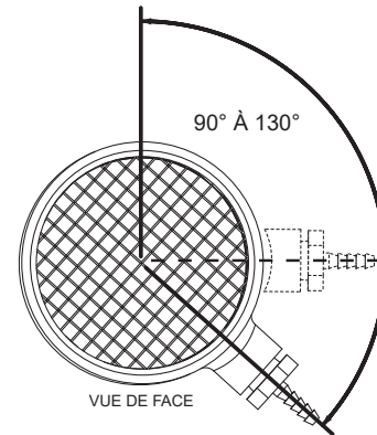
Figure 25. Orientation de l'embout cannelé de raccordement d'admission d'air
