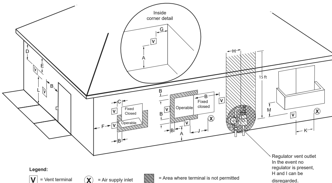
Figure 65. Évacuation directe murale utilisant l'air extérieur
