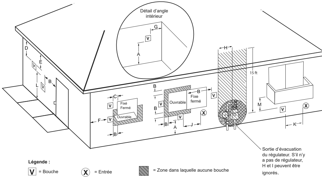
Figure 66. Évacuation autre qu'une évacuation directe murale utilisant l'air extérieur
