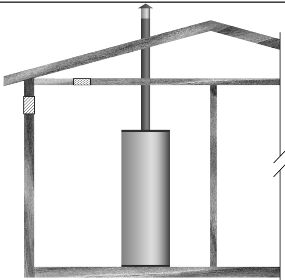
Figure 18. Air extérieur à travers une ouverture
