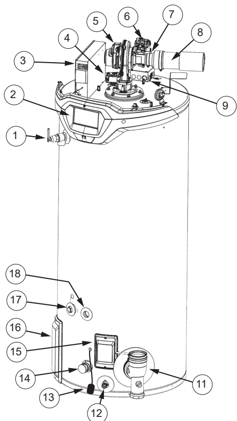
Figure 9. Composants du côté droit
