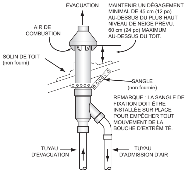
Figure 43. Extrémité concentrique - Installation verticale
