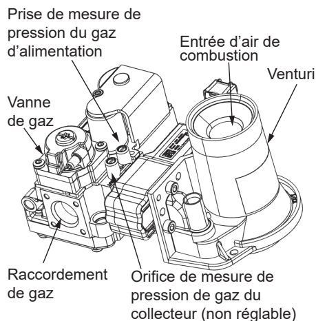
Figure 71. VK 100 gallons - Raccordement de la conduite d'arrivée de gaz
