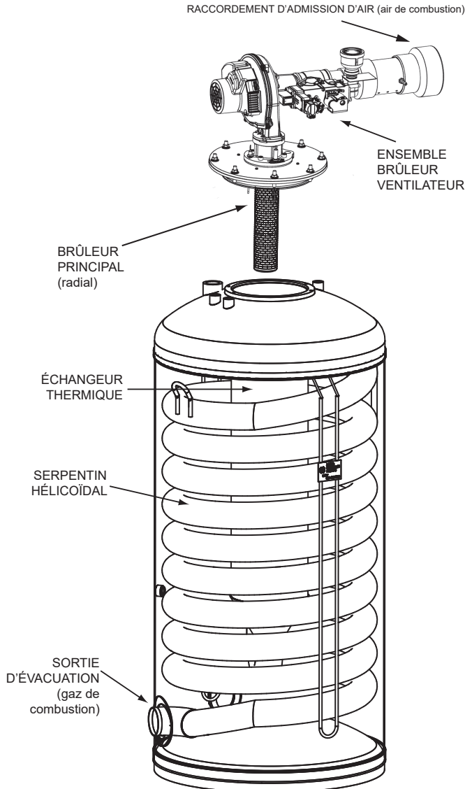
Figure 1. Composants fonctionnels
