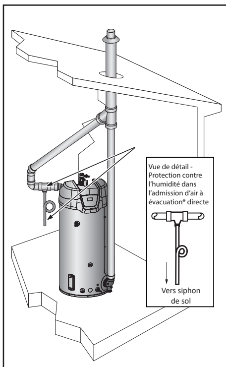
Figure 62. Évacuation directe concentrique verticale
