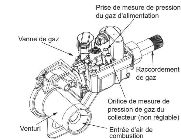
Figure 70. PX52 60 gallons - Raccordement de la conduite d'arrivée de gaz
