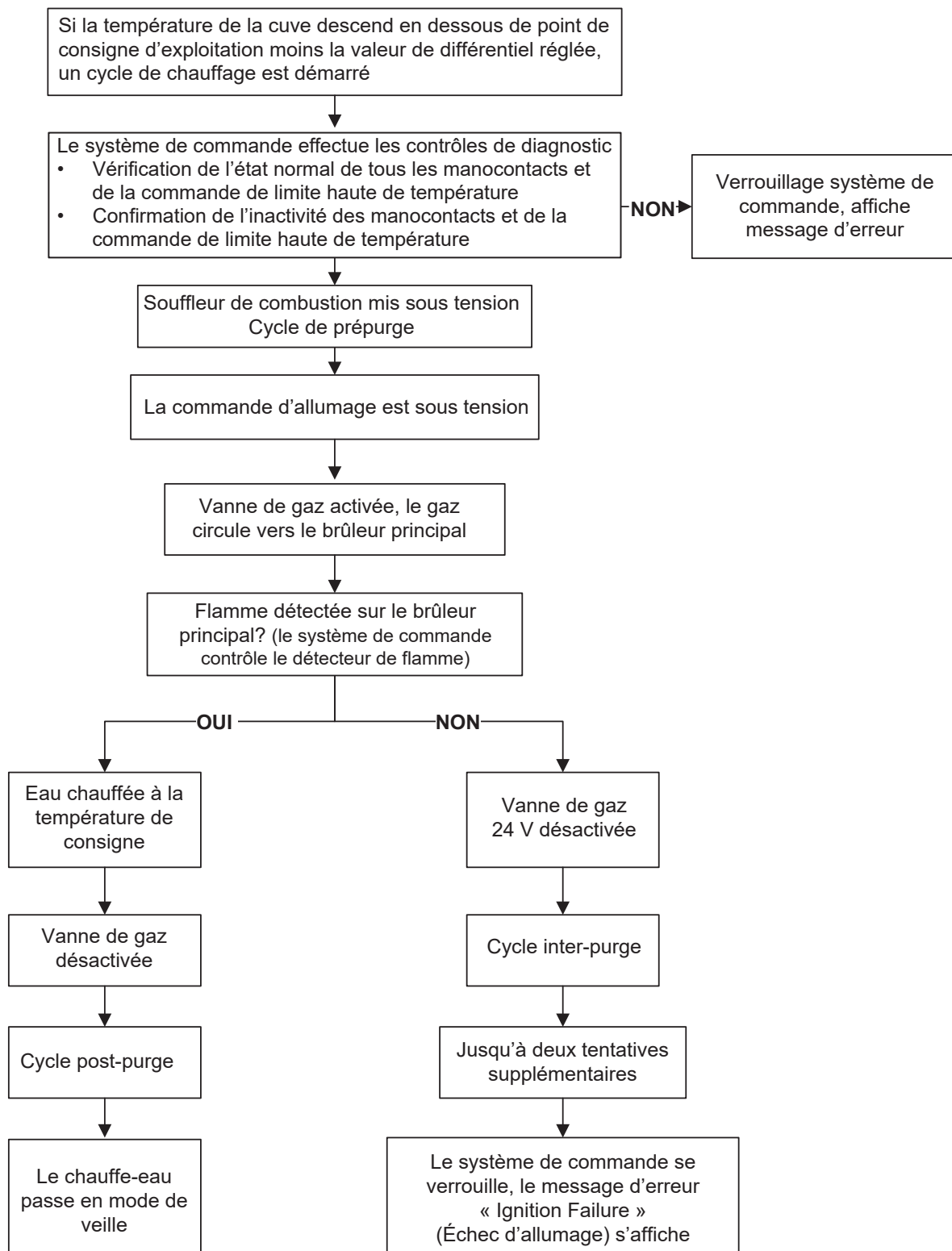
Figure 85. Séquence de fonctionnement
