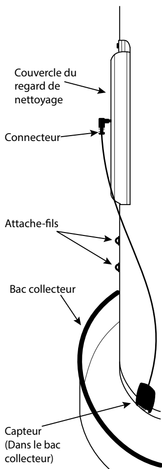
Figure 68. Installation du module de détection de fuite
