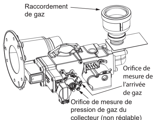
Figure 72. 119 gallons - Raccordement de la conduite d'arrivée de gaz
