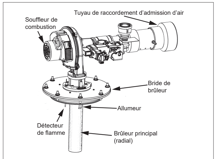
Figure 4. Ensemble souffleur-brûleur - 119 gallons
