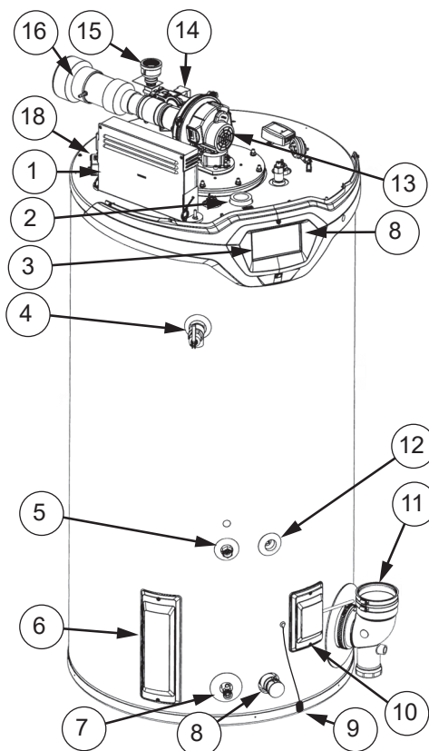
Figure 10. Côté gauche
