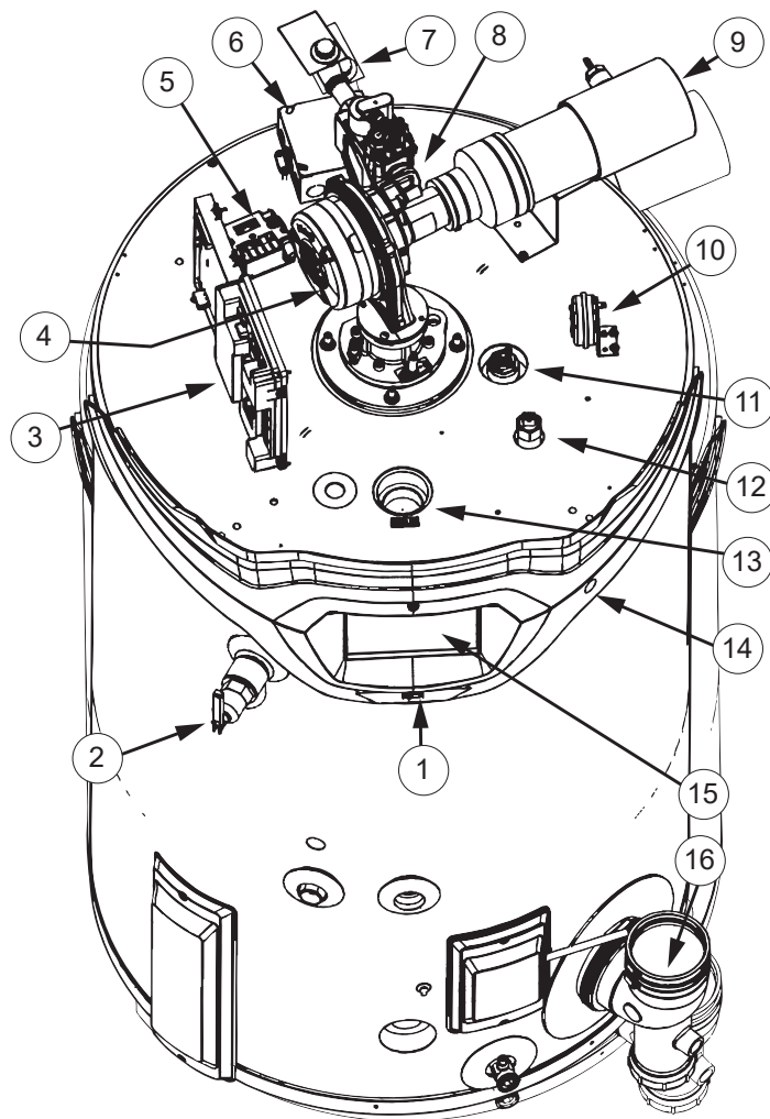
Figure 5. Vue de dessus, 60 gallons
