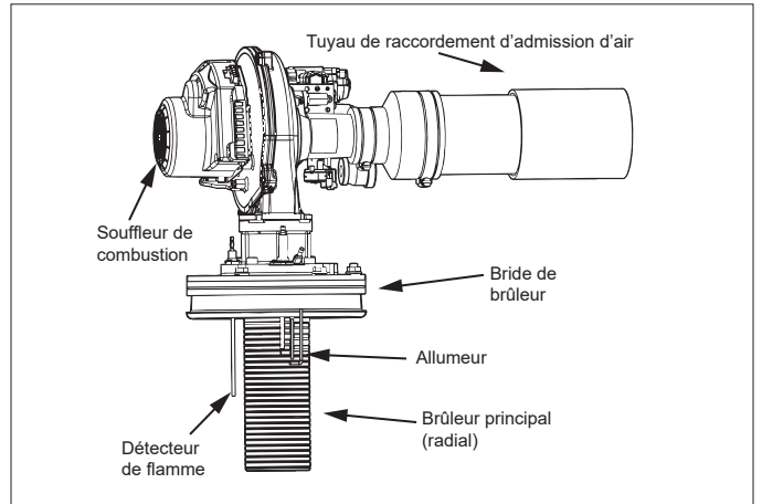
Figure 3. Ensemble souffleur-brûleur - 100 gallons
