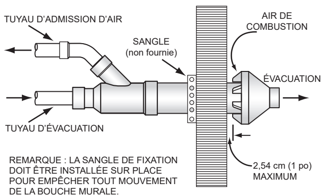
Figure 44. Extrémité concentrique - Installation murale
