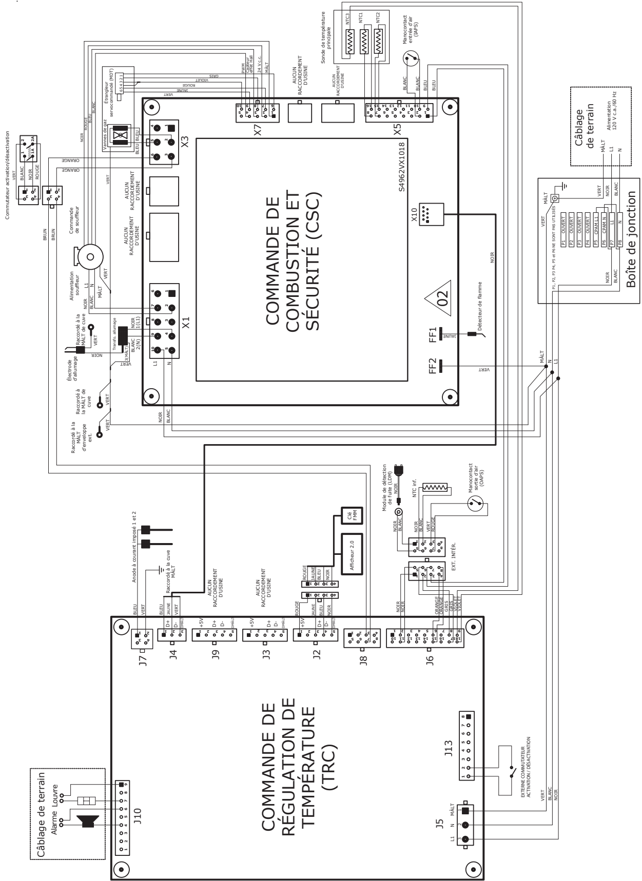
Figure 90. Modèles 100 gallons - Schéma de câblage de la commande de régulation de température et du contrôleur de combustion et de sécurité
