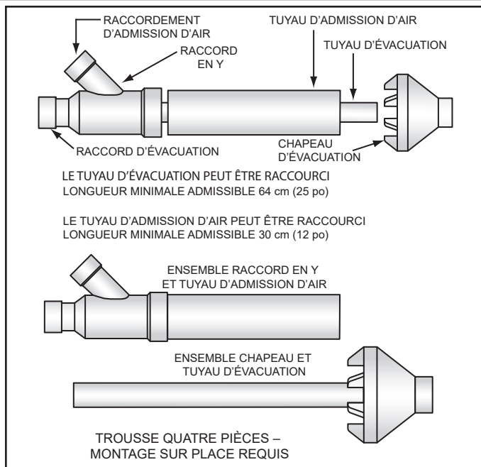
Figure 41. Nécessaire bouche d'extrémité concentrique - 60/100 gallons
