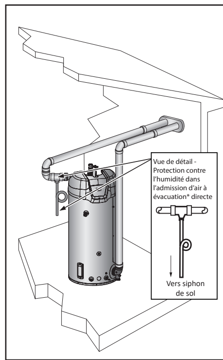
Figure 64. Évacuation directe compacte horizontale
