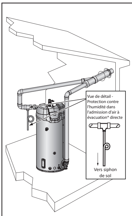
Figure 63. Évacuation directe concentrique horizontale
