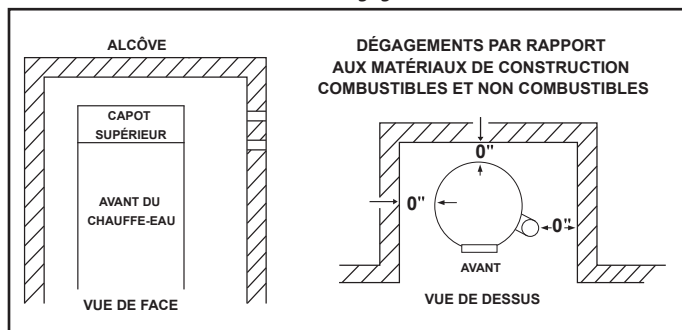
Figure 13. Dégagements
