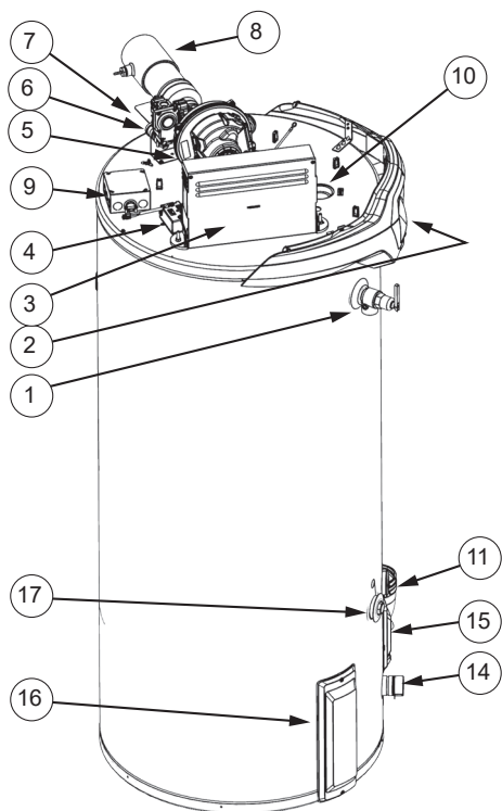
Figure 8. Composants du côté gauche
