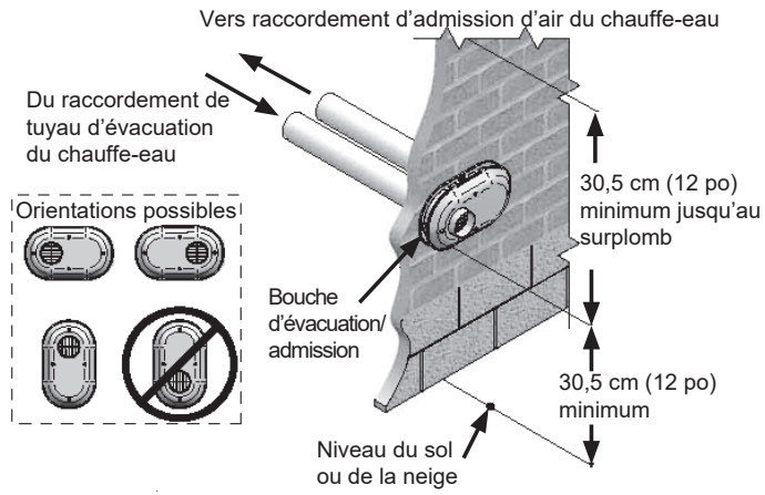
Figure 54. Flux d'entrée et d'évacuation dans les installations à bouche d'extrémité compacte
