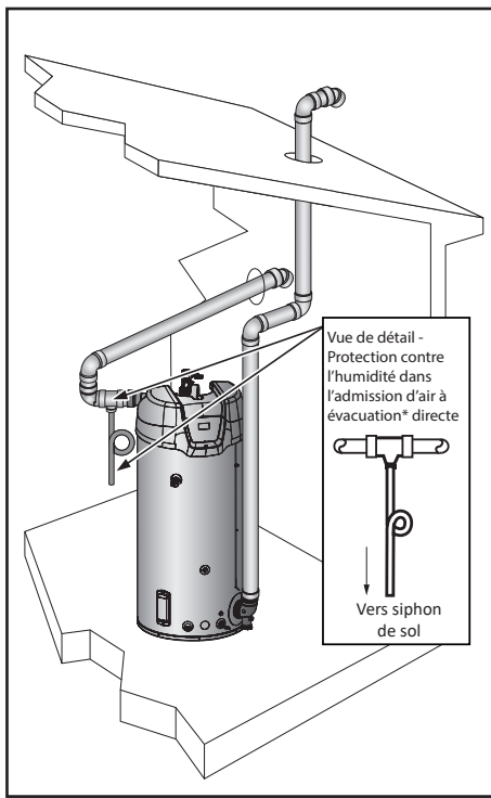
Figure 60. Évacuation directe, échappement vertical, admission horizontale
