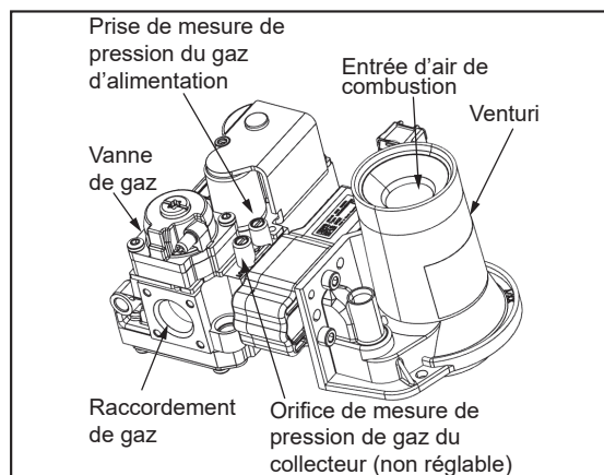
Figure 75. VK 100 gallons - Vanne de gaz
