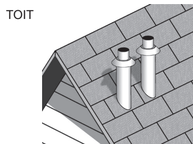
Figure 50. Deux bouches concentriques - Mur et toit
