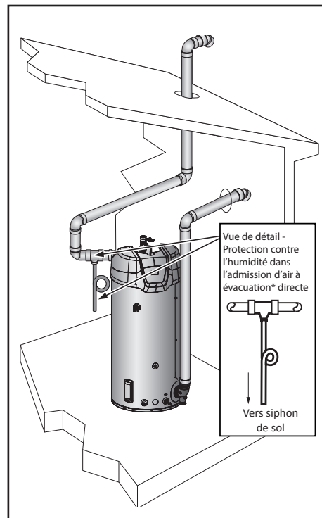
Figure 61. Évacuation directe, échappement horizontal, admission verticale
