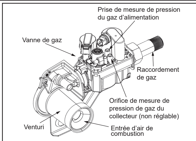
Figure 74. PX52 60 gallons - Vanne de gaz
