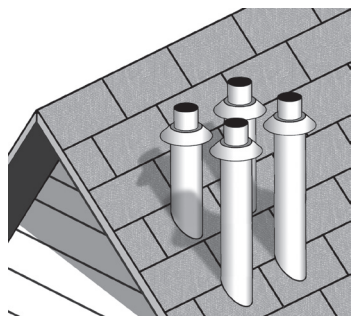
Figure 51. Quatre bouches concentriques - Mur et toit
