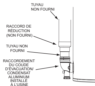
Figure 31. Raccordement d'évacuation des gaz de combustion
