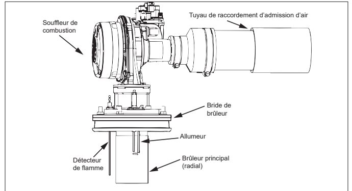
Figure 2. Ensemble souffleur-brûleur - 60 gallons
