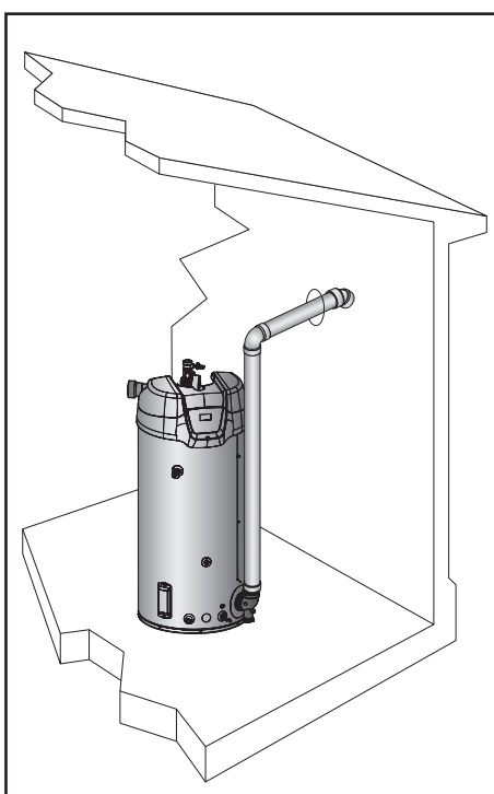
Figure 57. Évacuation mécanique horizontale
