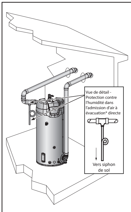
Figure 59. Évacuation directe horizontale
