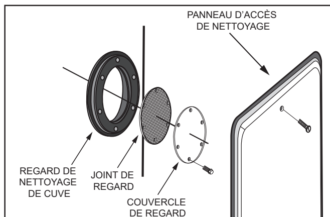
Figure 81. Regard de nettoyage
