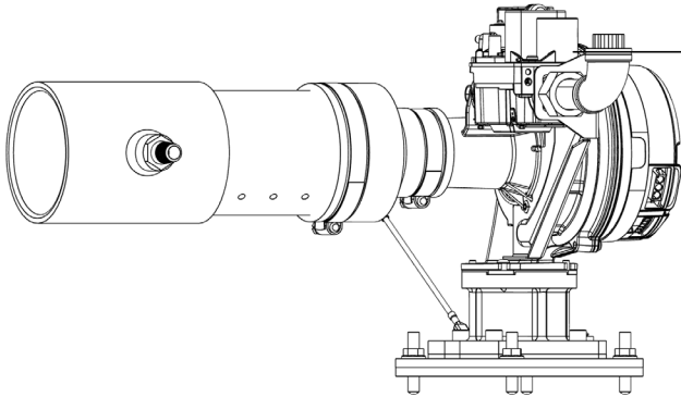
Figure 22. Raccordement d'admission d'air
