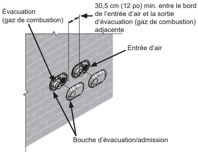
Figure 55. Dégagement entre plusieurs bouches d'extrémité compactes
