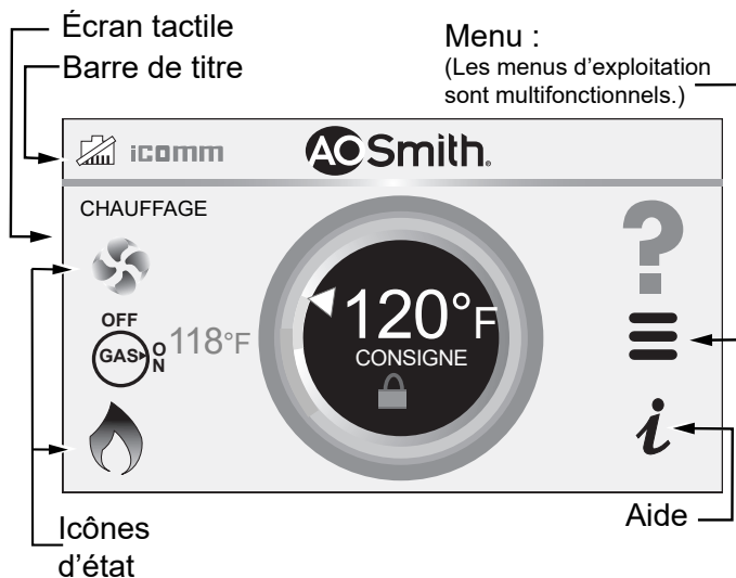
Figure 80. Écran d'accueil du module d'interface utilisateur (MIU)
