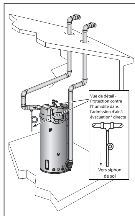
Figure 58. Évacuation directe verticale
