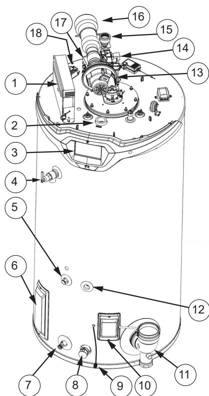
Figure 11. Côté droit
