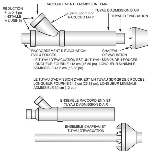
Figure 42. Nécessaire bouche d'extrémité concentrique - 119 gallons
