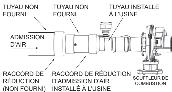
Figure 34. Raccordement d'admission d'air
