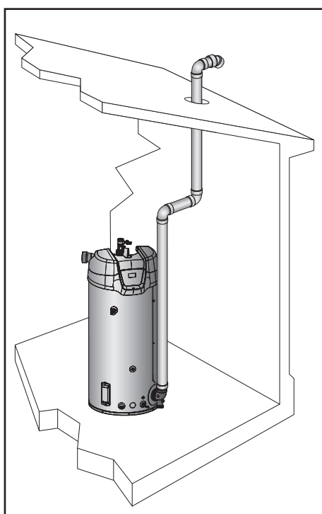
Figure 56. Évacuation mécanique verticale
