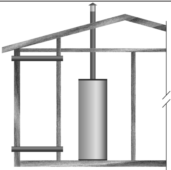
Figure 19. Air extérieur à travers deux conduits horizontaux
