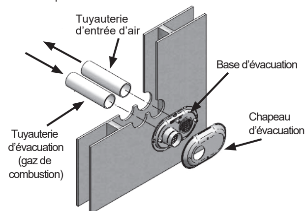
Figure 53. Flux d'entrée et d'évacuation dans les installations à extrémité compacte
