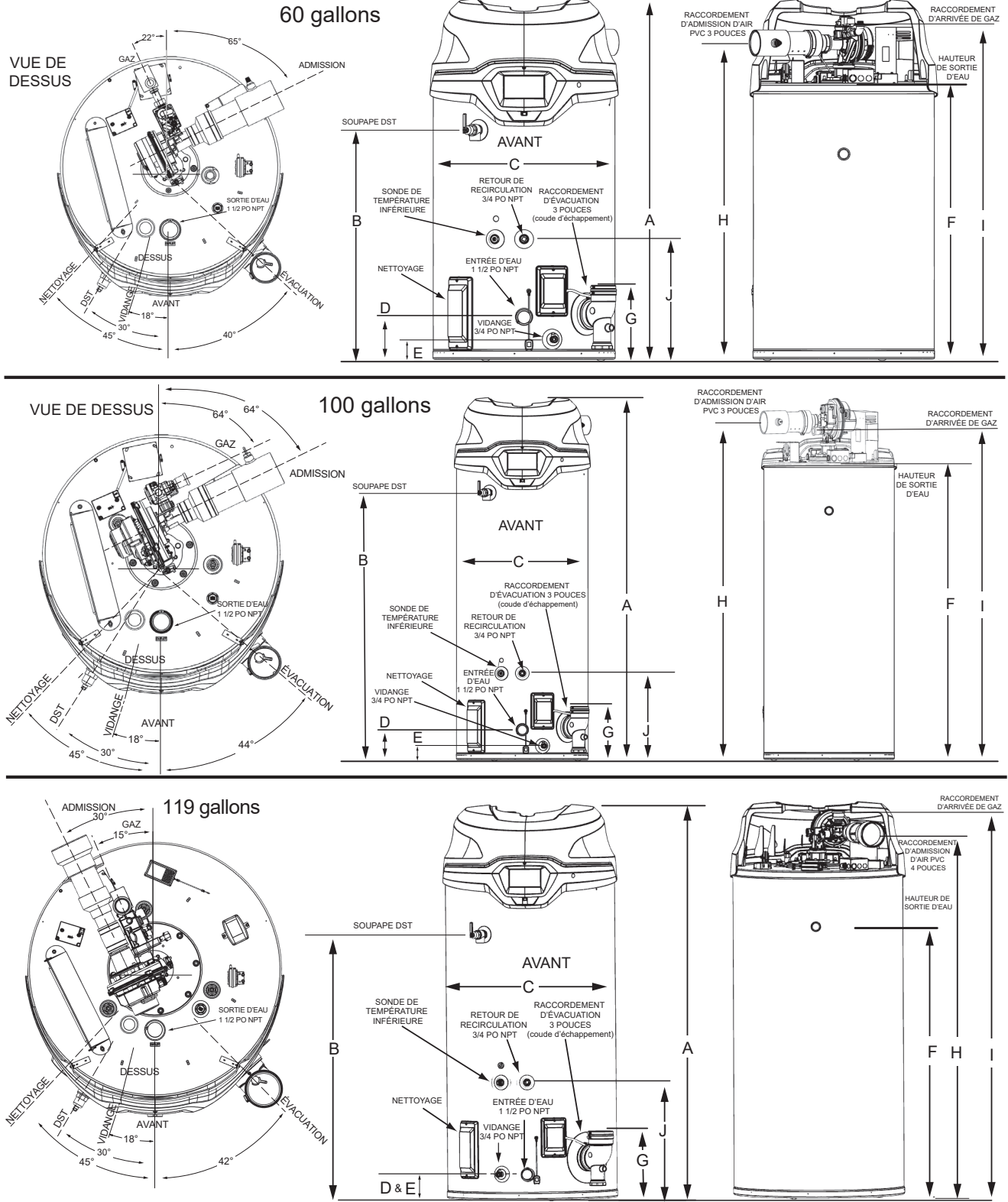
Figure 12. Dimensions de mise en place des conduites
