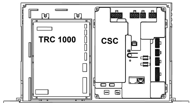
Figure 79. Composants du système de commande
