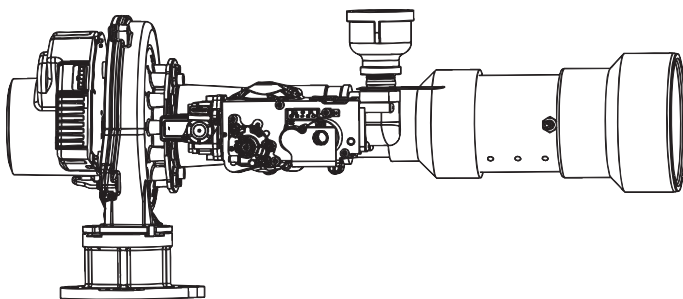
Figure 24. Raccordement d'admission d'air (100 gallons)
