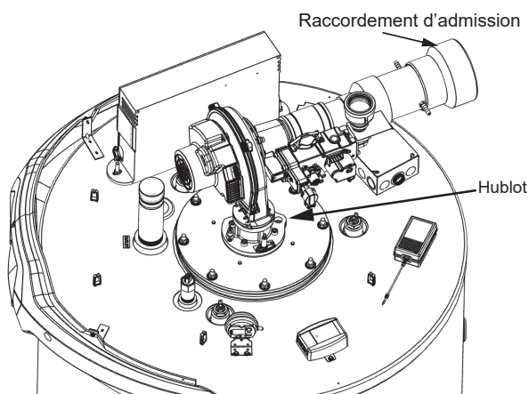
Figure 82. Emplacement du hublot
