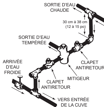
Figure 14. Mitigeur
