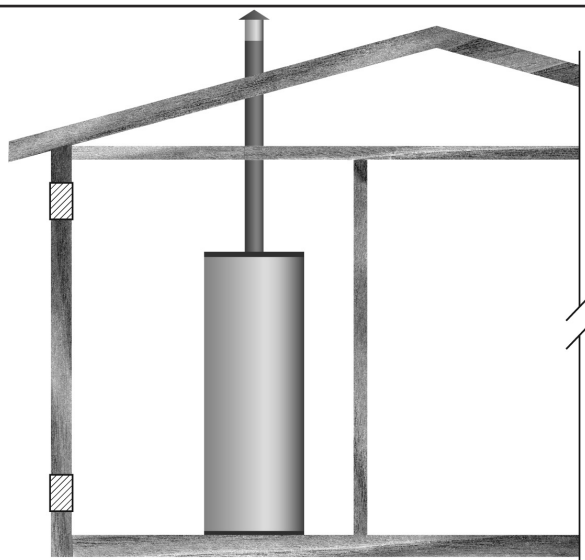
Figure 17. Air extérieur à travers deux ouvertures
