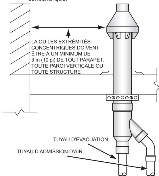
Figure 40. Extrémité concentrique - Dégagement sur toit plat à parapet
