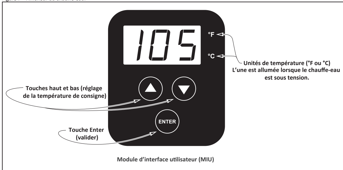
Figure 7 - Afficheur du chauffe-eau.
