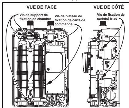
Figure 30 - Emplacement des vis de fixation.
