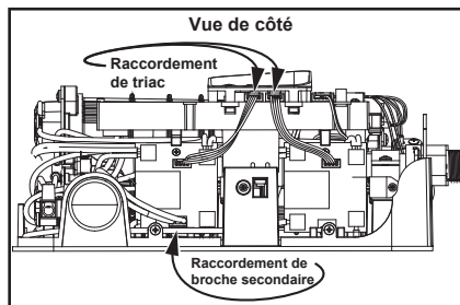
Figure 48 - Triac(s) et raccordement de broche secondaire.
