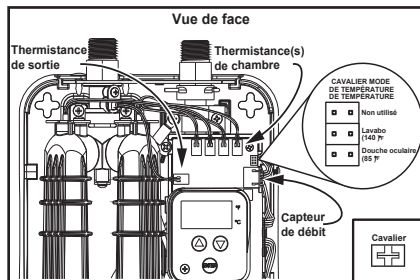
Figure 47 - Thermistances, capteur de débit et cavalier.
