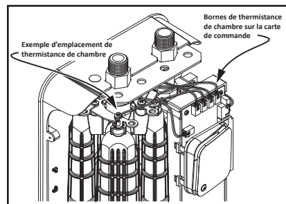
Figure 25 - Emplacement de la thermistance de chambre.
