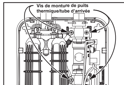
Figure 31 - Vis de montage de puits thermique/tube d'arrivée.
