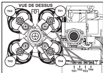
Figure 29 - Configuration des câbles de thermistance.
