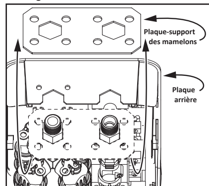
Figure 32 - Démontage de la plaque-support des mamelons.
