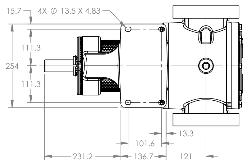
VIEW A-A
