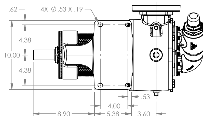
VIEW A-A
