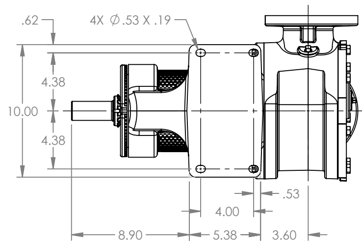
VIEW A-A
