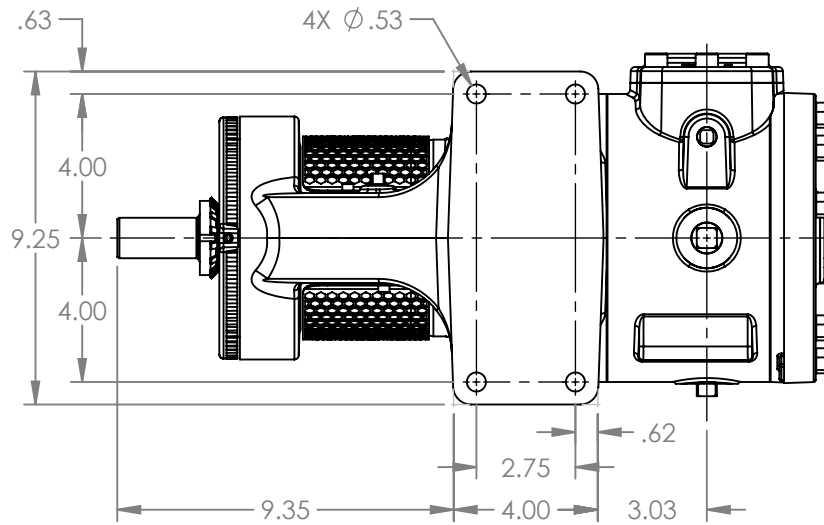
VIEW A-A
