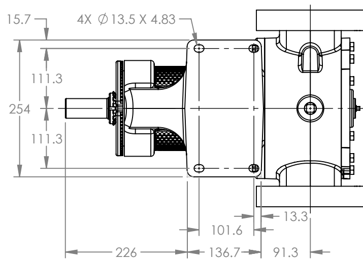
VIEW A-A
