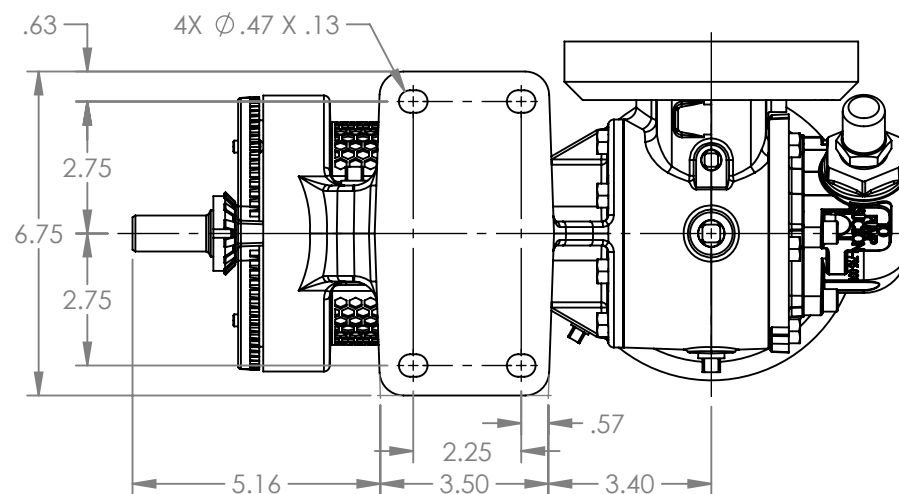
VIEW A-A
