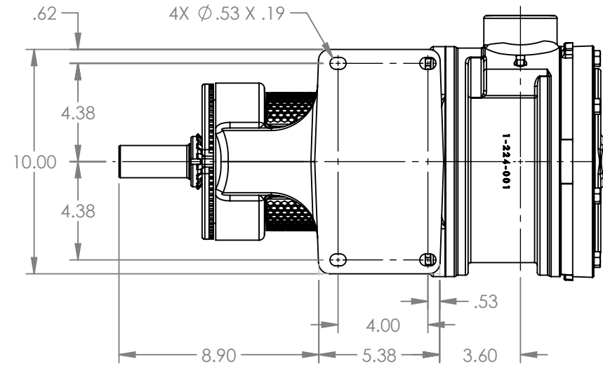
VIEW A-A
