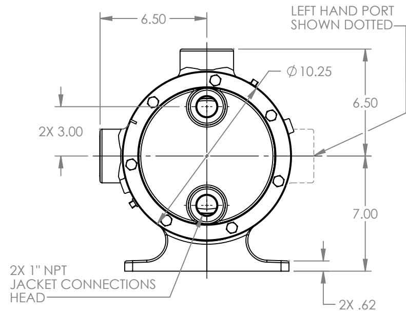
VIEW A-A
