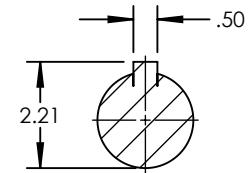
SECTION A-A SCALE 1 : 4
