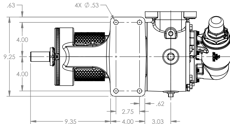
VIEW A-A
