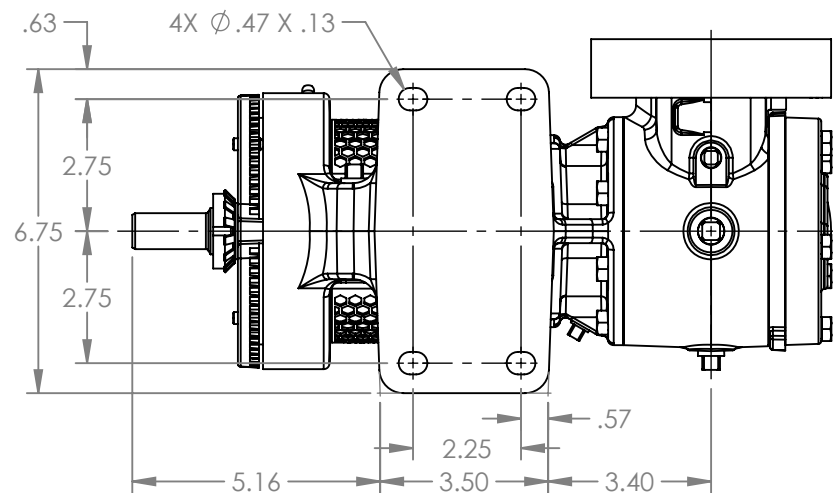
VIEW A-A
