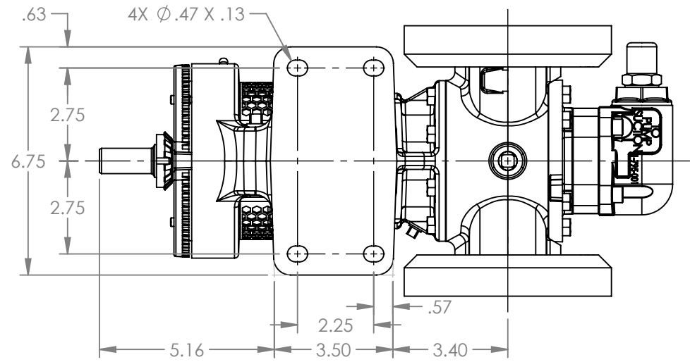
VIEW A-A
