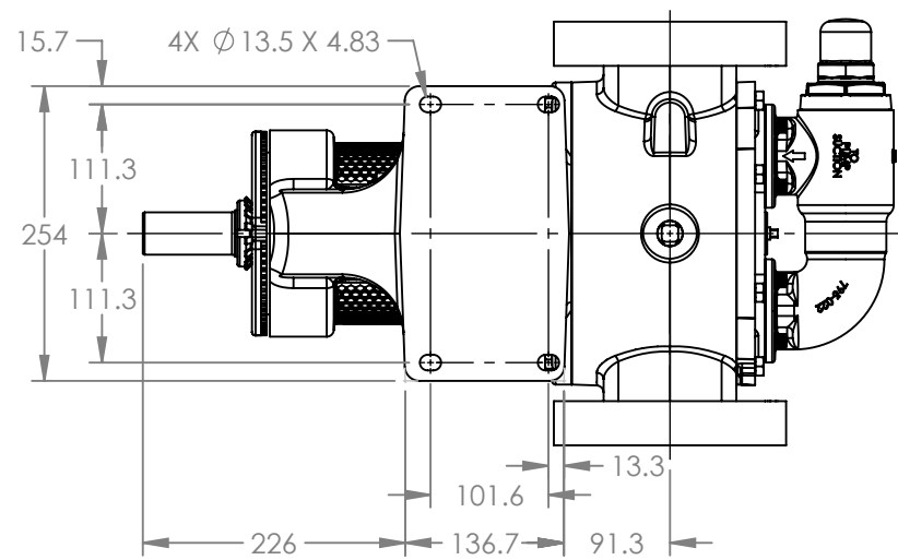
VIEW A-A
