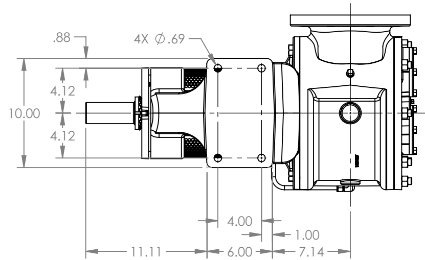
VIEW A-A
