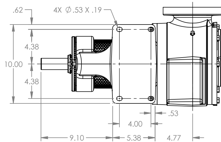
VIEW A-A
