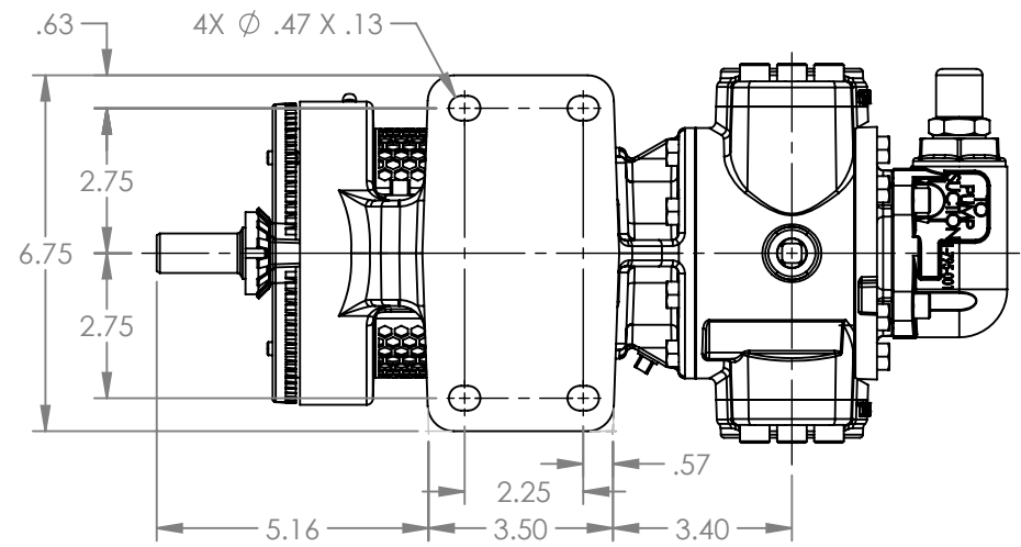
VIEW A-A
