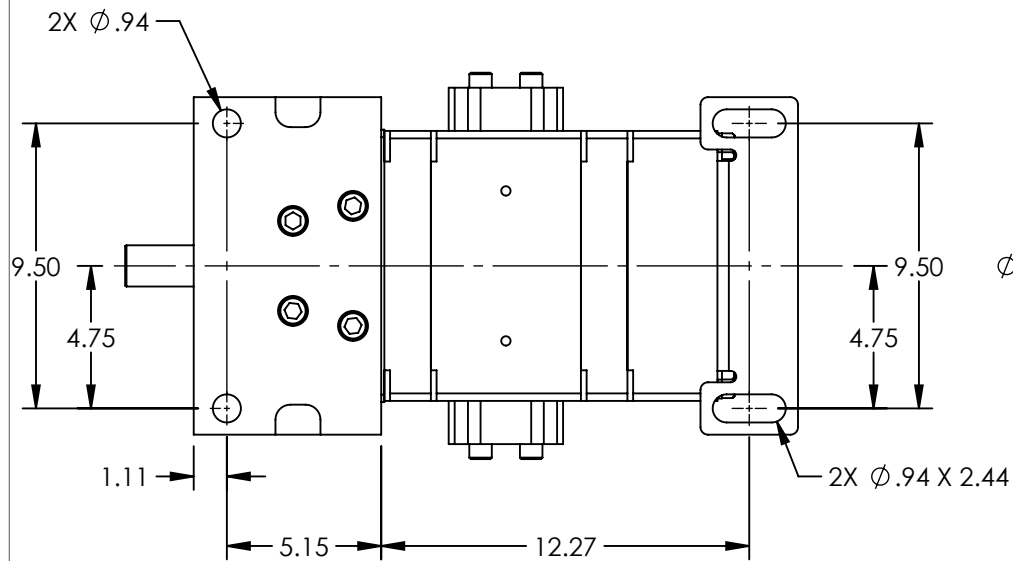
VIEW A-A
